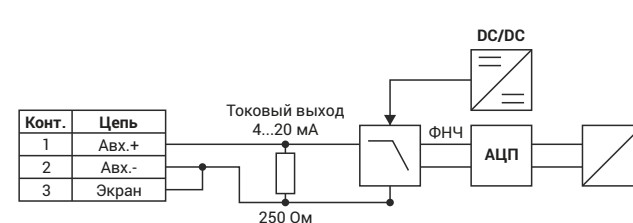
Структурная схема аналогового входа
