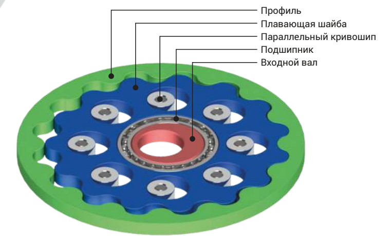
Циклоидальная передача
