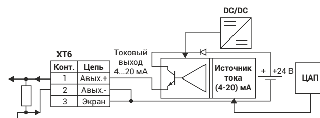
Структурная схема аналогового выхода
