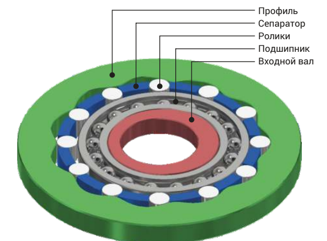
Волновая передача с промежуточными телами качения
