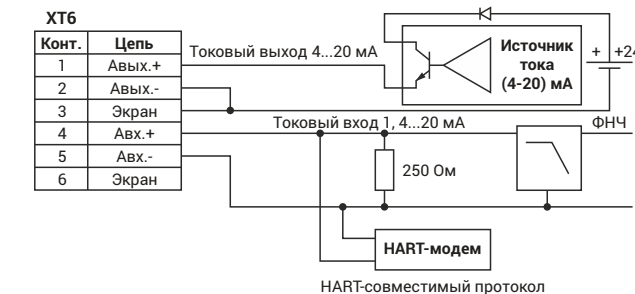
Структурная схема интерфейса HART
