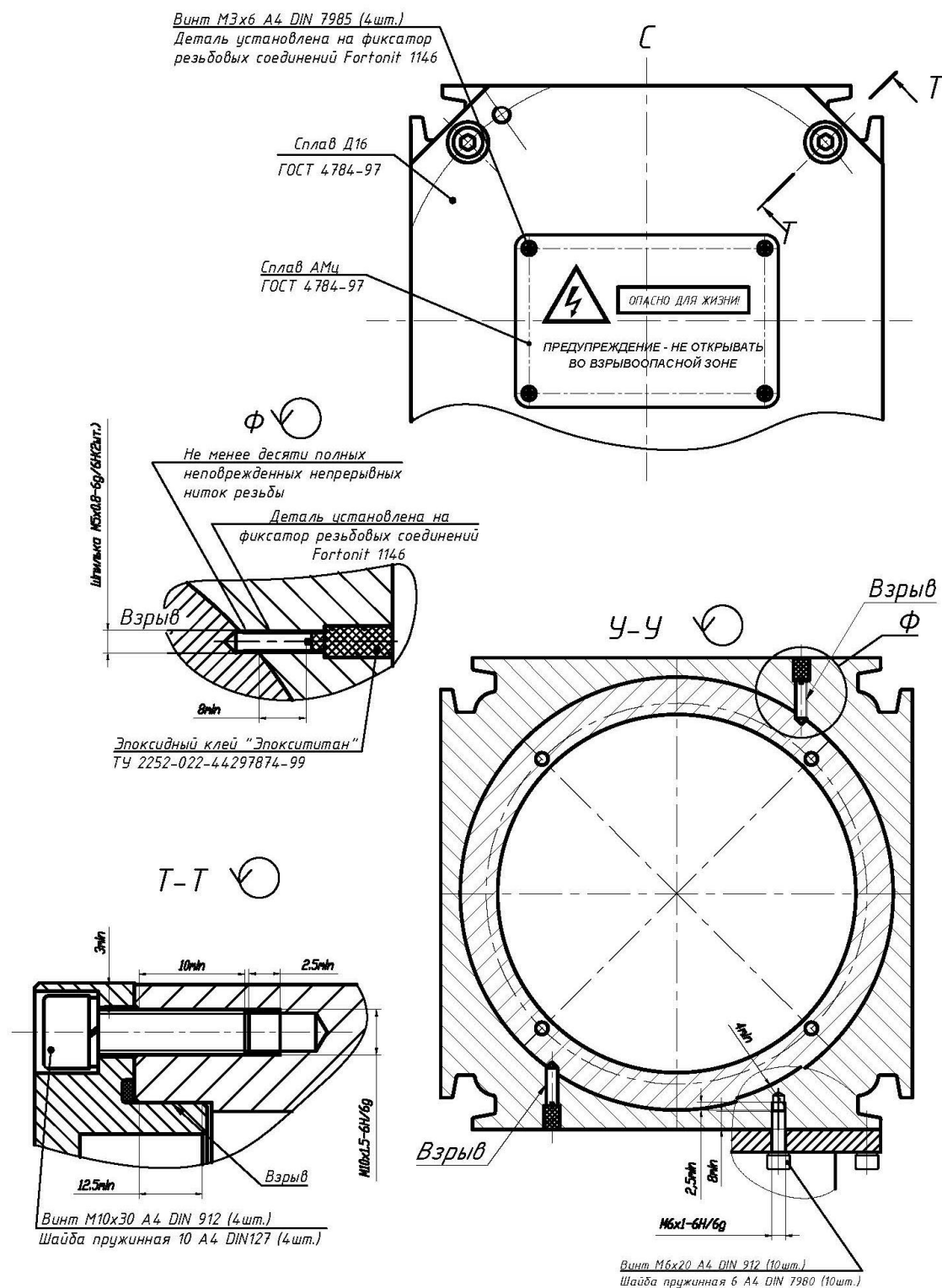
Рисунок Д.1 (продолжение) – Чертеж средств взрывозащиты РЭМТЭК конструктивного исполнения "94"
