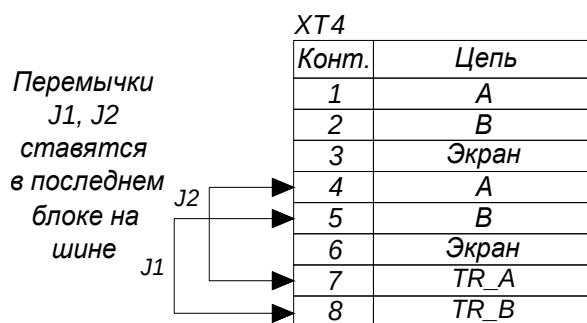
Рисунок 15а – Схема подключения с помощью перемычек
