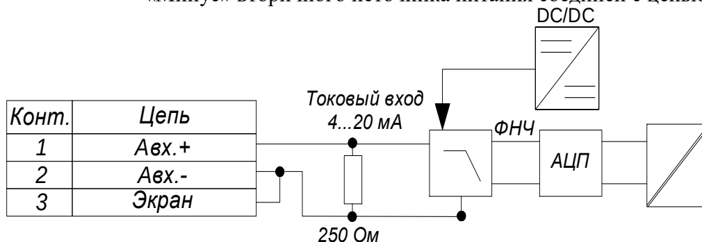
Рисунок 11 – Структурная схема аналогового входа
