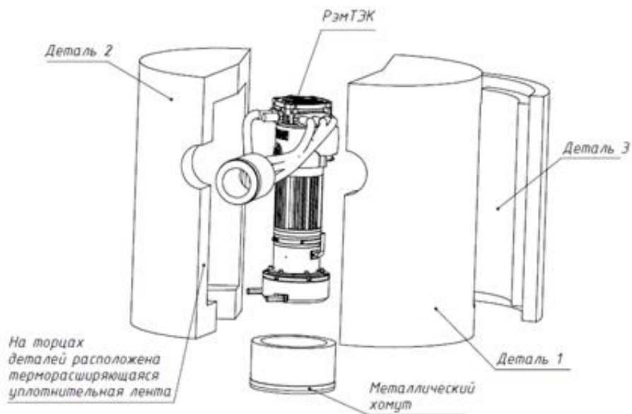
Рисунок 26 – Схема 1
