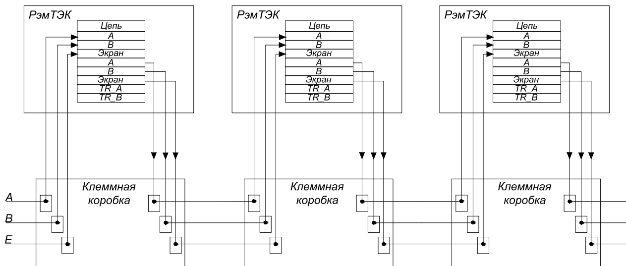
Рисунок 14 – Схема 1
