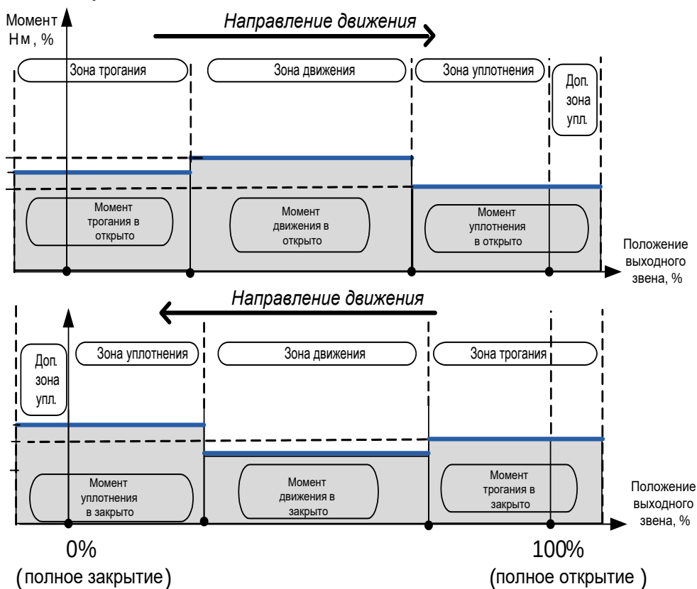
Рисунок 31 – Диаграмма движения запирающего элемента арматуры
