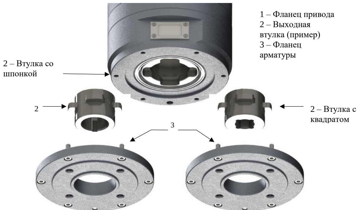
Рисунок 20 - Схема установки РэмТЭК многооборотного и неполнооборотного исполнения
