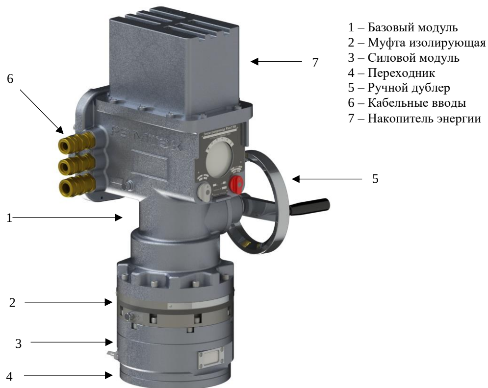
Рисунок 4 – Составные части электроприводов РэмТЭК 91, 95
