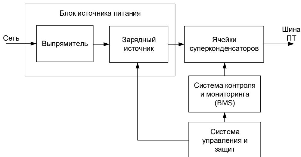
Рисунок 16а – Структурная схема энергонакопителя для 94 конструктивного исполнения
