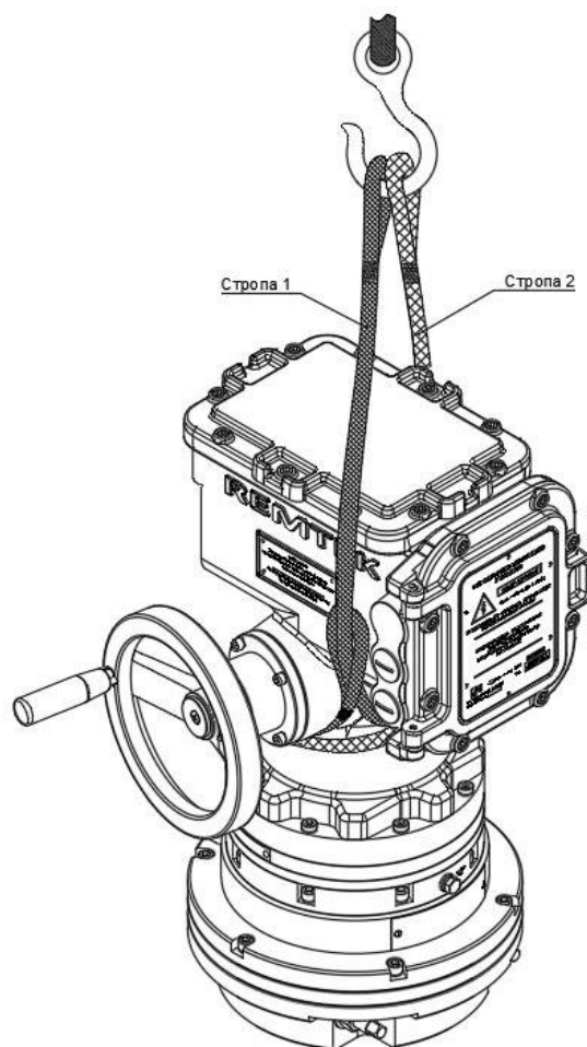
Рисунок 19а – Рекомендуемая схема строповки
