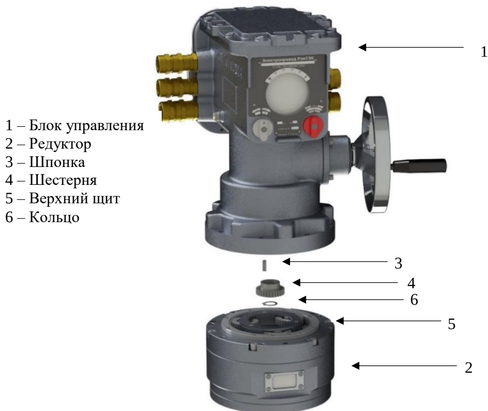
Рисунок 35 – Порядок замены редуктора
