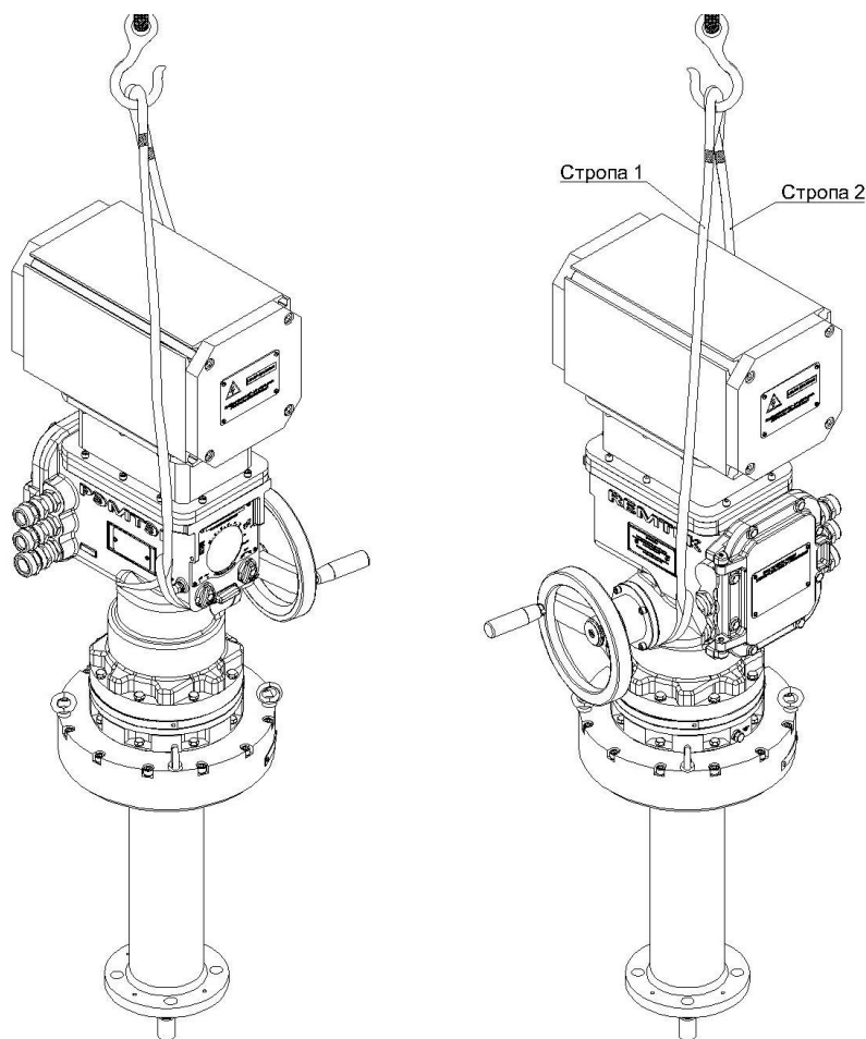
Рисунок 196 – Схемы строповки электропривода Л.65000.50 конструктивного исполнения «9400»
