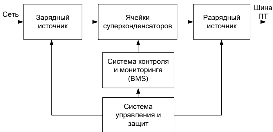
Рисунок 16 – Структурная схема энергонакопителя для 91,95 конструктивного исполнения
