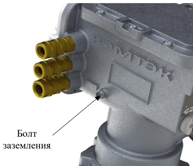
Рисунок 23 - Заземление электропривода
