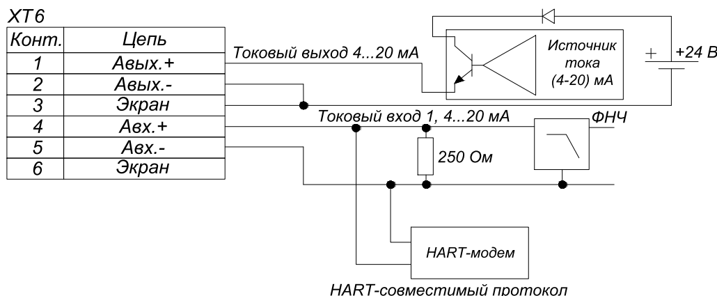
Рисунок 15в – Структурная схема подключения HART-интерфейса
