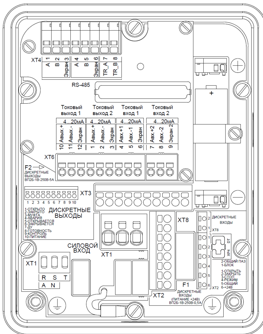
Рисунок 25 - Внешний вид бокса подключения
