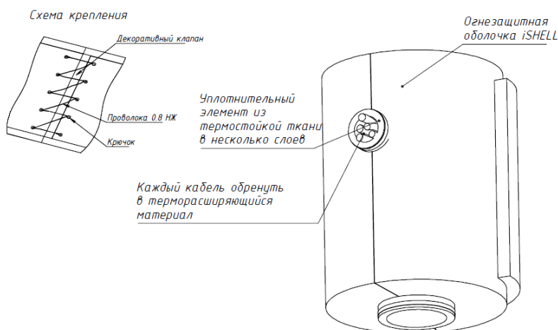
Рисунок 27 – Схема 2
