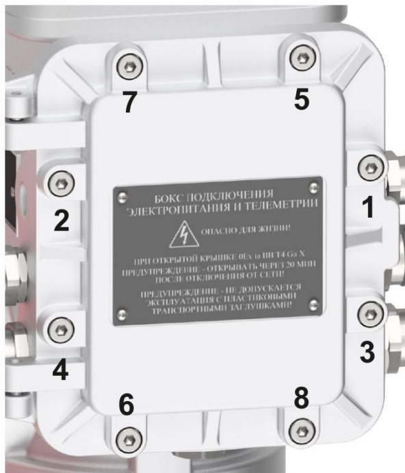
Рисунок 25а - Расположение болтов крепления крышки
