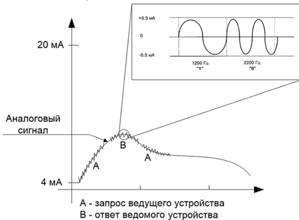
Рисунок 156 – Кодирование HART-сигнала
