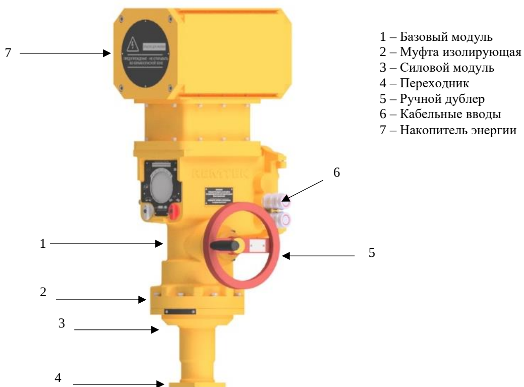
Рисунок 4а – Составные части электропривода РэмТЭК 94
