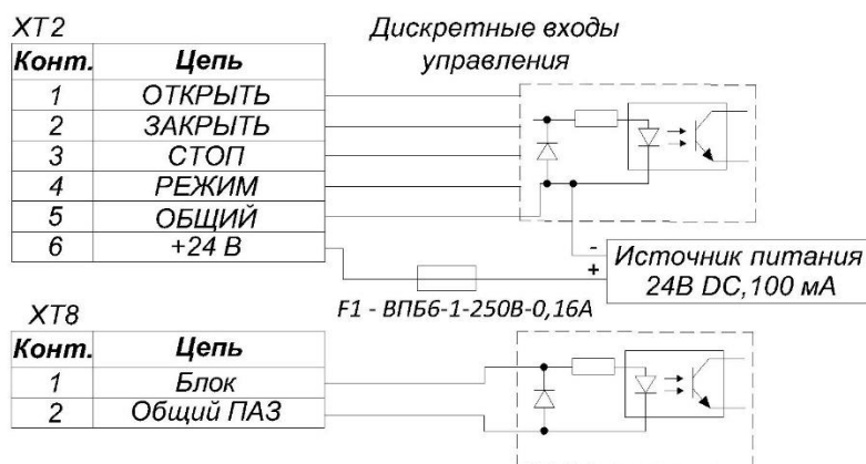
Рисунок 7 – Структурная схема дискретного входа
