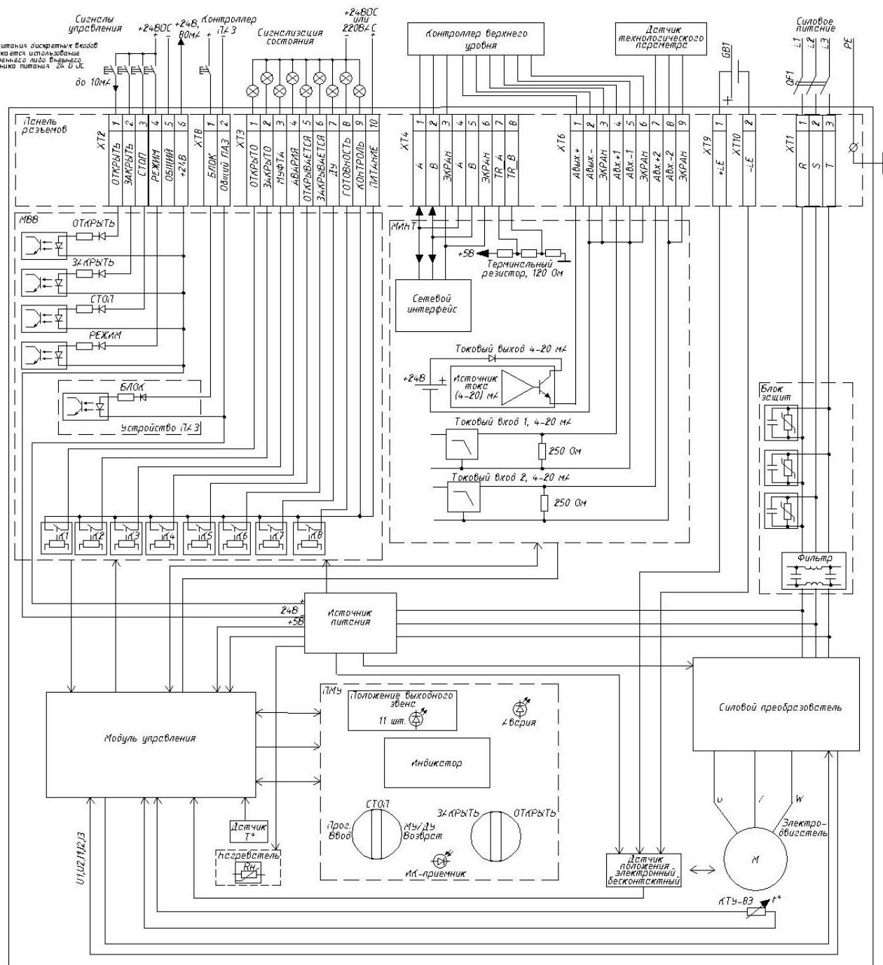
Рисунок Е.2 – Схема электрическая функциональная РэмТЭК при питании от трехфазной цепи переменного тока напряжением 400 В частотой 50 Гц
