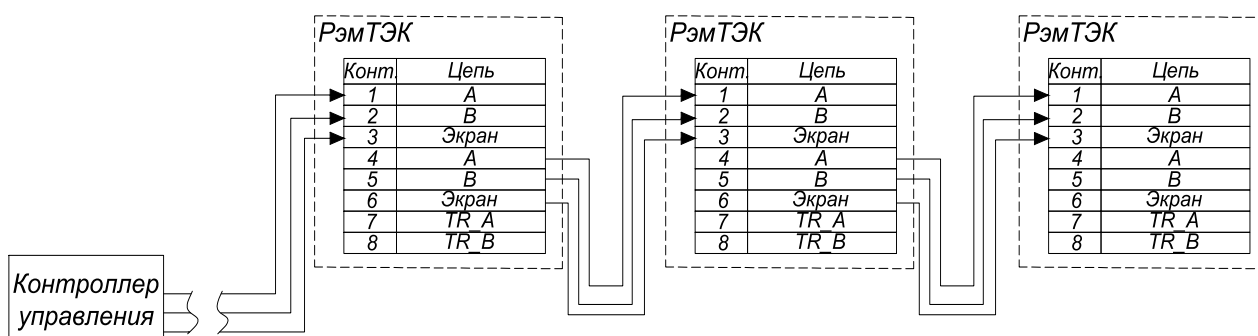
Рисунок 15 – Схема 2
