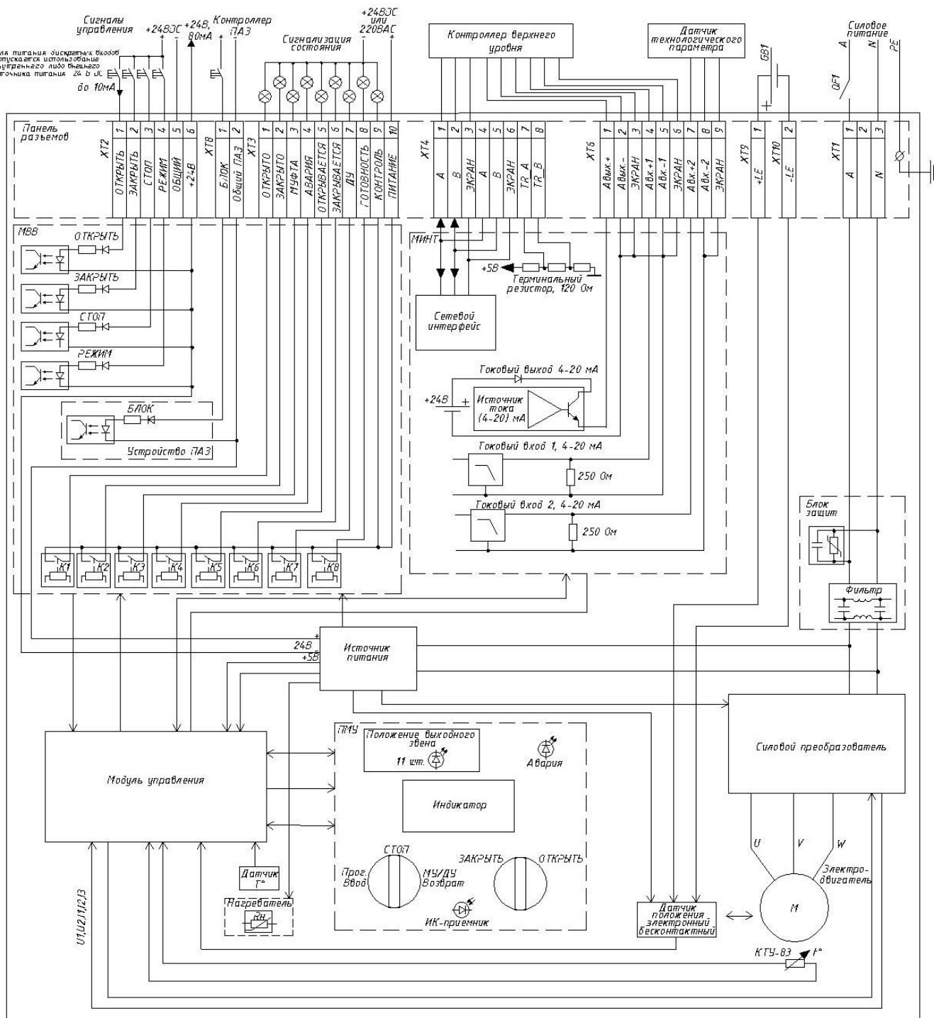
Рисунок Е.1 – Схема электрическая функциональная РэмТЭК при питании от однофазной цепи переменного тока напряжением 230 В частотой 50 Гц
