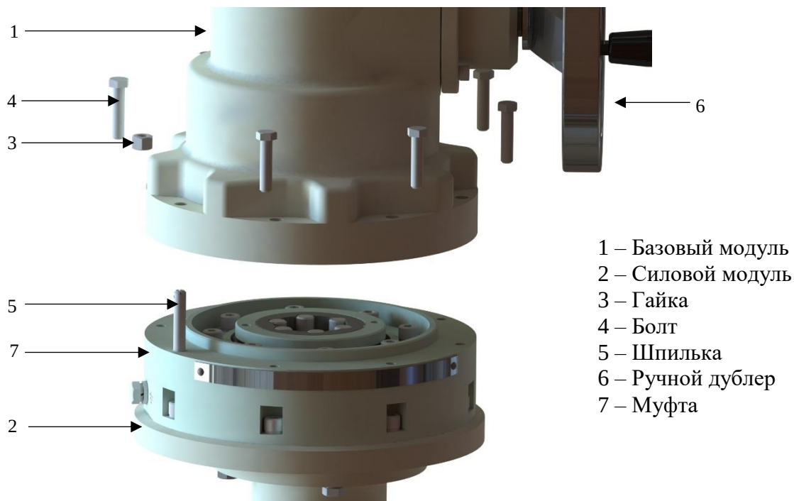
Рисунок 22 - Поворот БМ относительно редуктора
