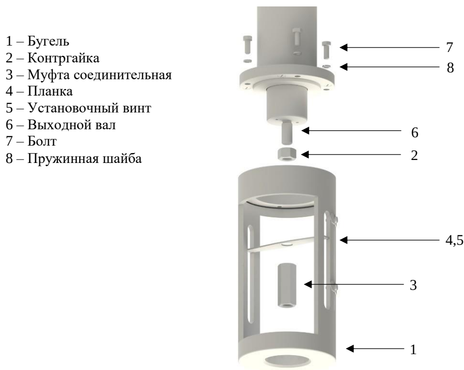
Рисунок 21 - Схема установки РэмТЭК прямоходного исполнения
