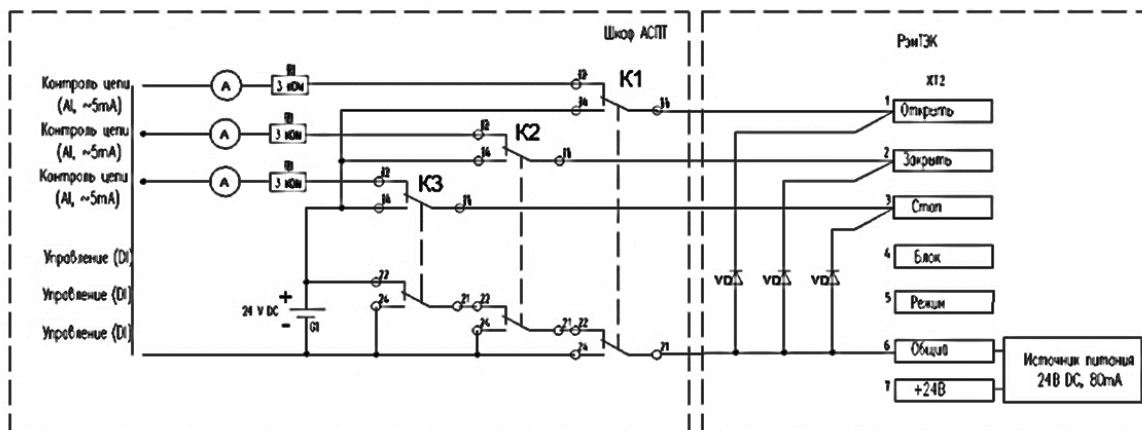
Рисунок 9а – Схема тестирования дискретных входов
