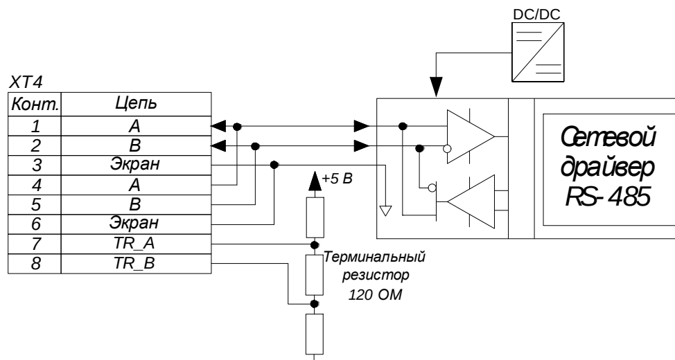
Рисунок 13 – Структурная схема интерфейса RS-485
