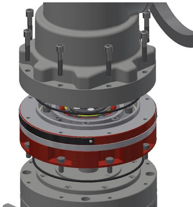
Рисунок 36 – Порядок замены редуктора
