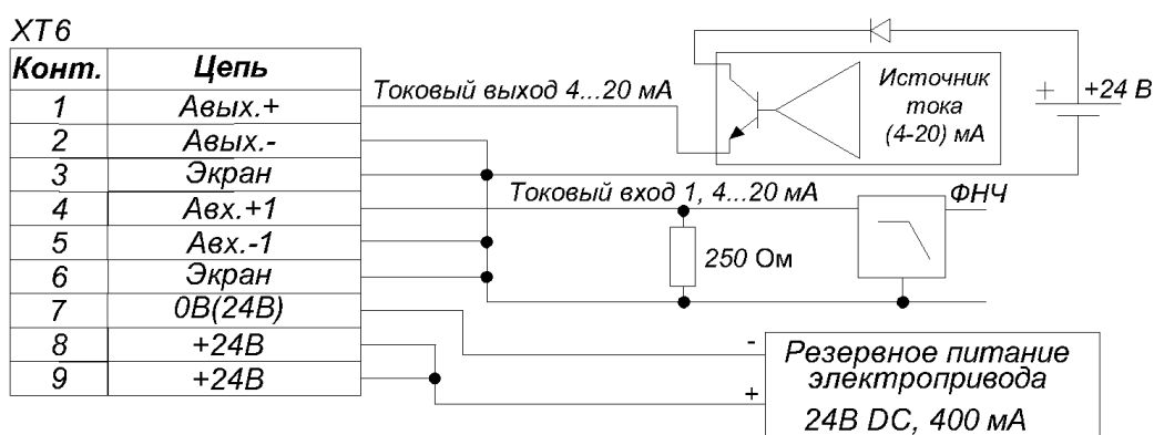
Рисунок 18 – Схема подключения
