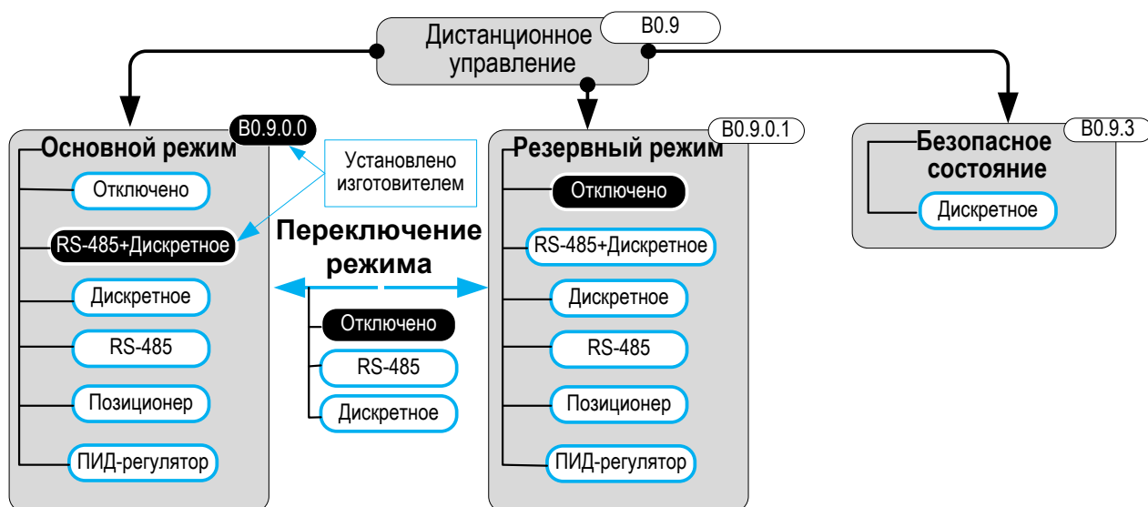
Рисунок 30 – Настройка режима работы по ДУ
