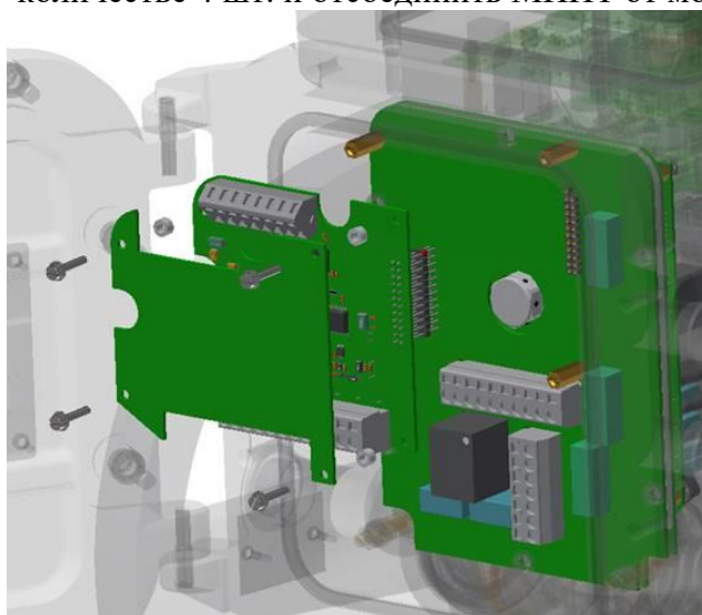
Рисунок 37 - Замена МИНТ
