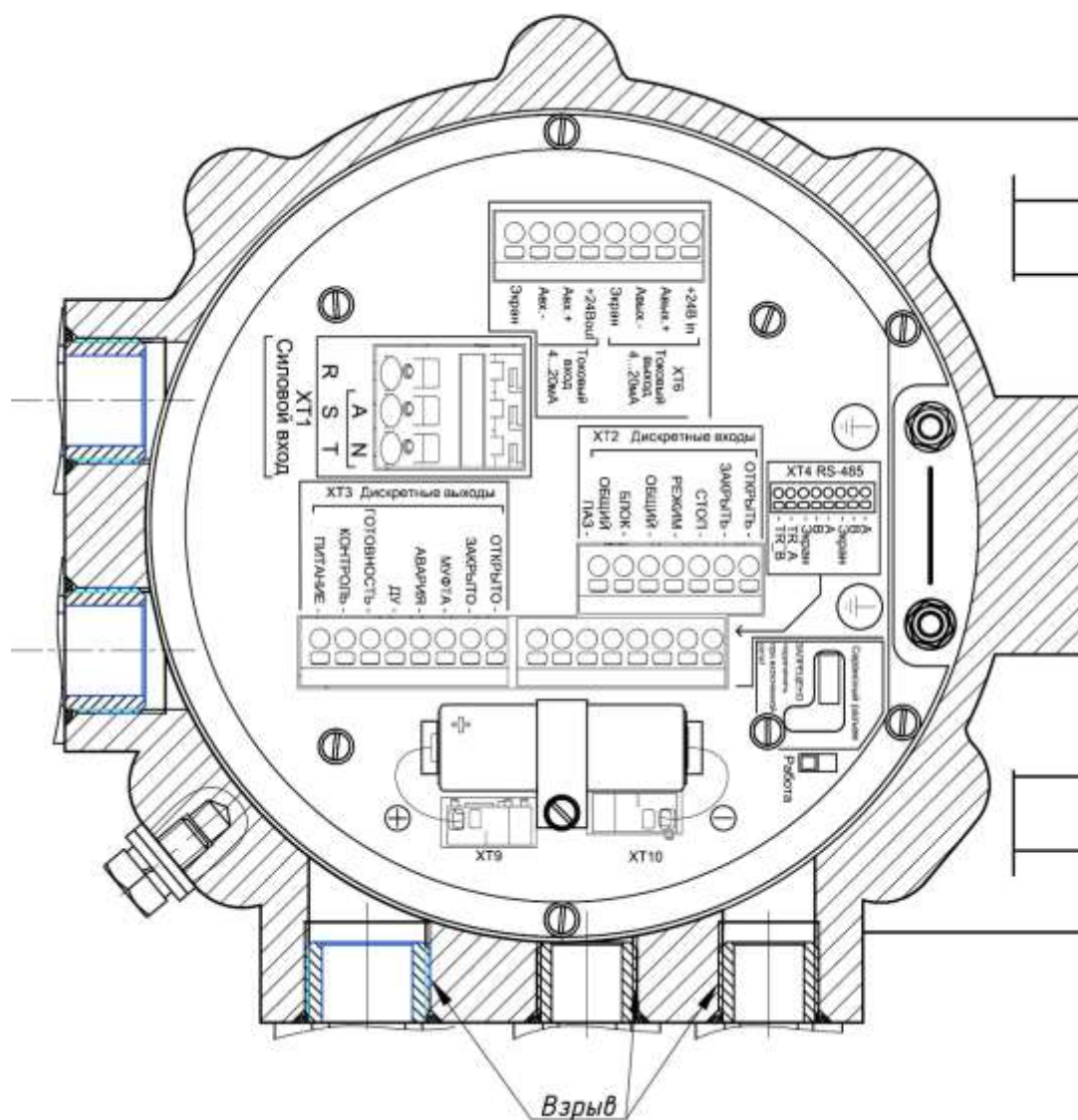
Рисунок 19 – Внешний вид бокса подключения РэмТЭК-VS конструктивного исполнения «83» (для модификации «51» по интерфейсным сигналам)
