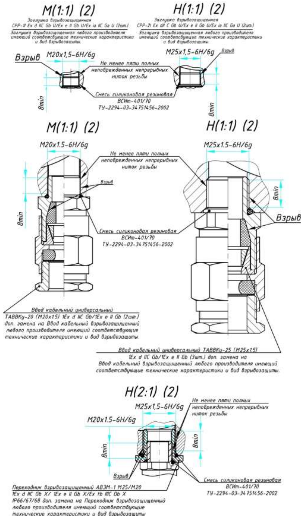
Рисунок Д.1 – Чертеж средств взрывозащиты РэмТЭК-VS (Лист 5)
