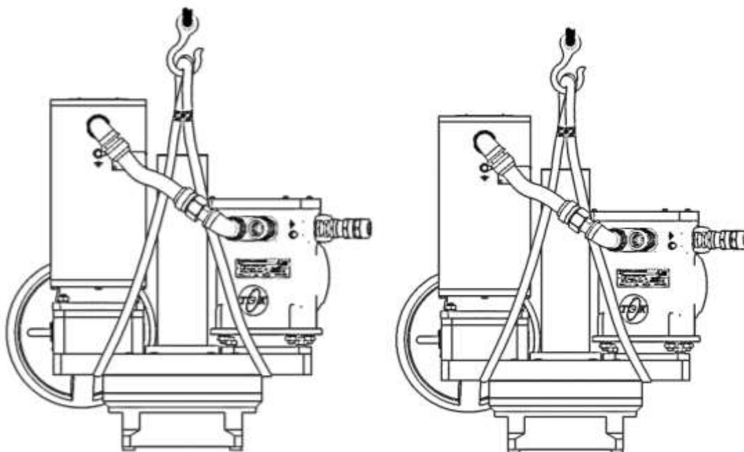
Рисунок 13 – Схема строповки (вариант 1)
