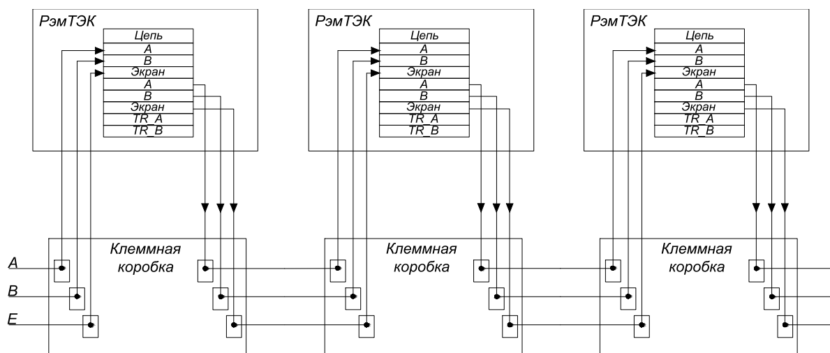
Рисунок 10 – Схема № 1 соединения электроприводов
