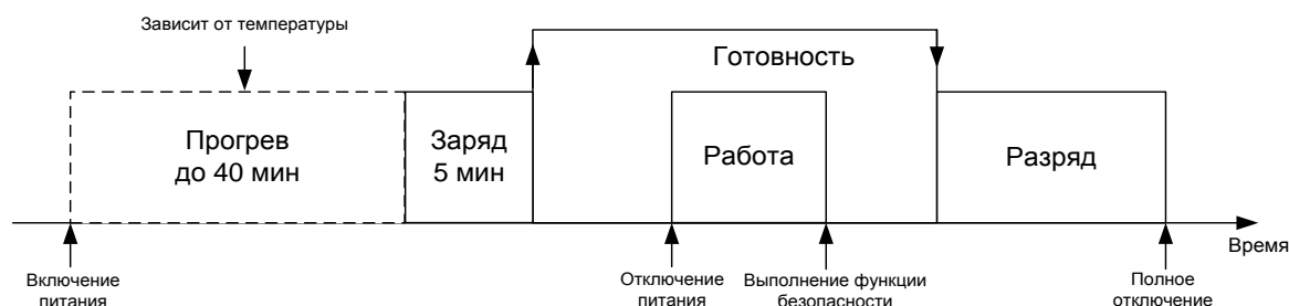
Рисунок 17 – Режимы работы накопителя Накопитель обеспечивает несколько режимов работы:
