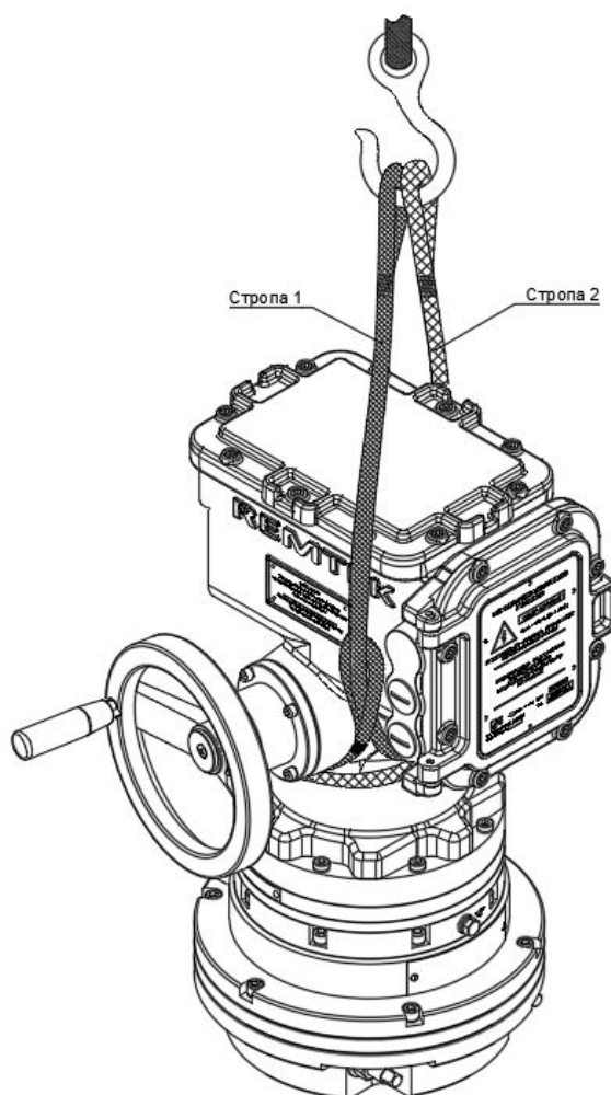
Рисунок 19 – Рекомендуемая схема строповки
