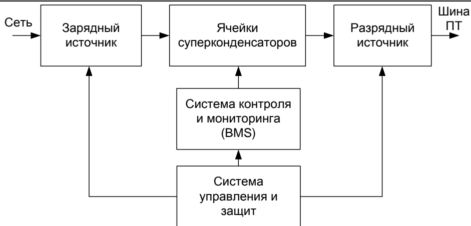
Рисунок 16 – Структурная схема энергоаккумулятора для 91,95 конструктивного исполнения
