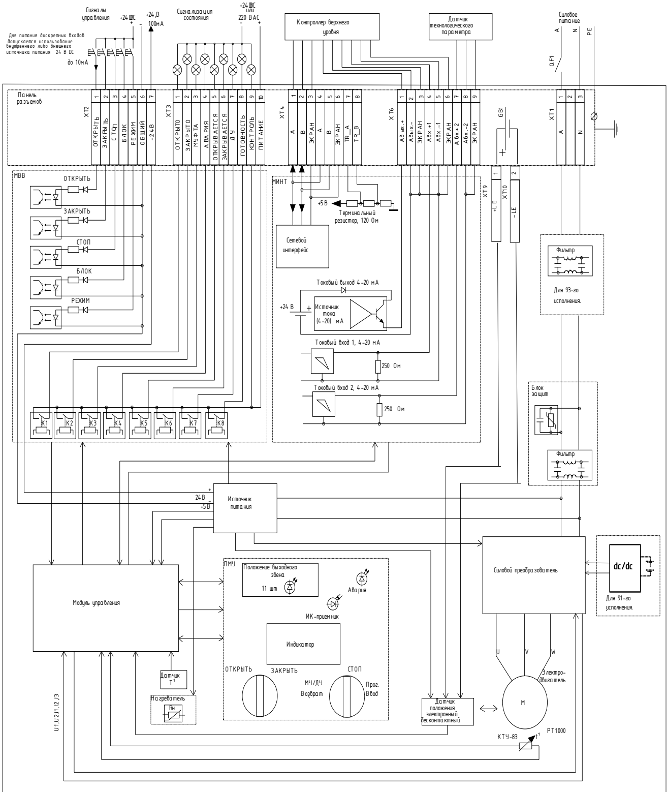
Рисунок Е.1 – Схема электрическая функциональная РэмТЭК при питании от однофазной цепи переменного тока напряжением 230 В частотой 50 Гц
