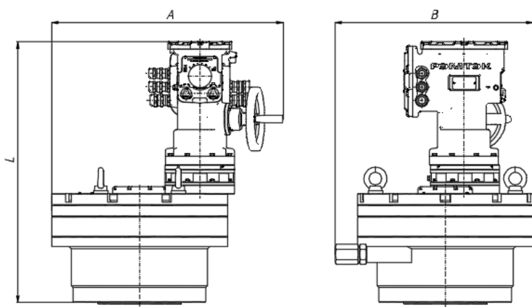
Рисунок И.4 – Габаритные размеры привода РэмТЭК.П.16000.ХХ - РэмТЭК.П.90000.ХХ
