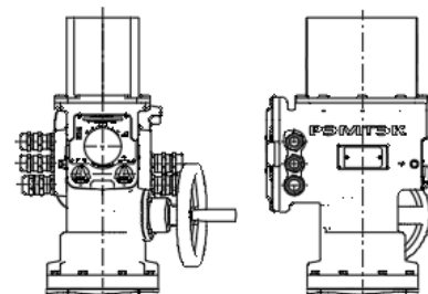
Рис.2 Исполнения 9100,9200,9300
