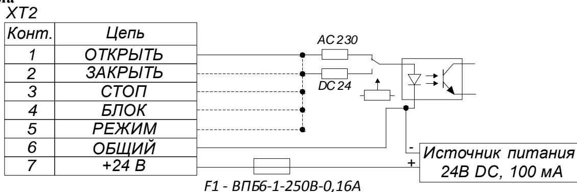
Рисунок 7 – Структурная схема дискретного входа
