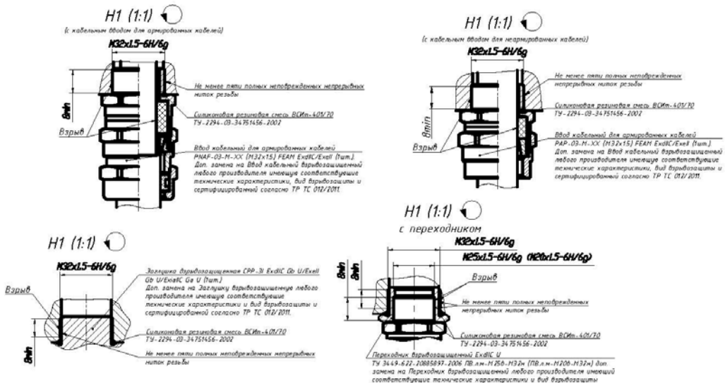
Рисунок Д.1 – Чертеж средств взрывозащиты РэмТЭК конструктивного исполнения "95"
