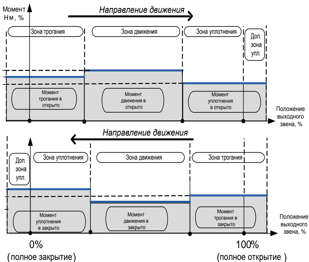
Рисунок 31 – Диаграмма движения запирающего элемента арматуры
