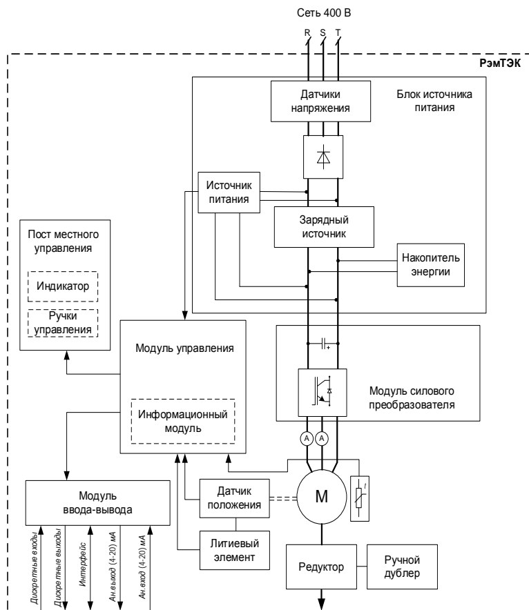
Рисунок 5 – Функциональная схема Базового модуля для электроприводов 91, 95 конструктивного исполнения
