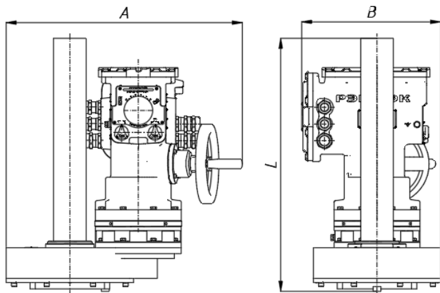
Рисунок И.2 – Габаритные размеры приводов РэмТЭК.М.300.ХХ - РэмТЭК.М.1000.ХХ
