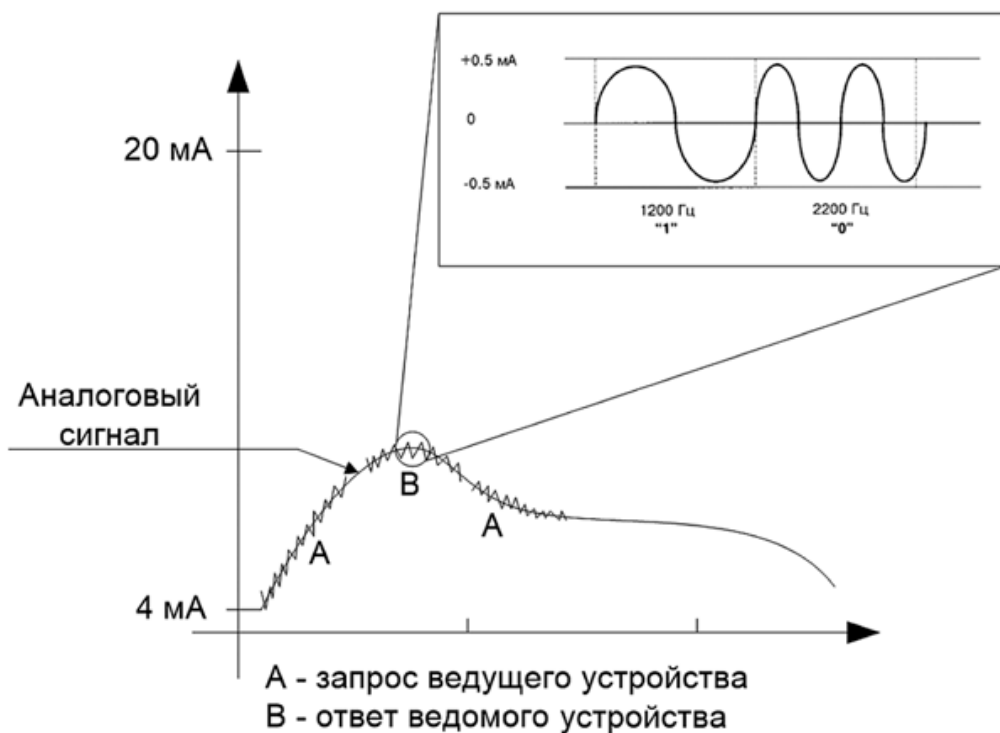
Рисунок 15а – Кодирование HART-сигнала
