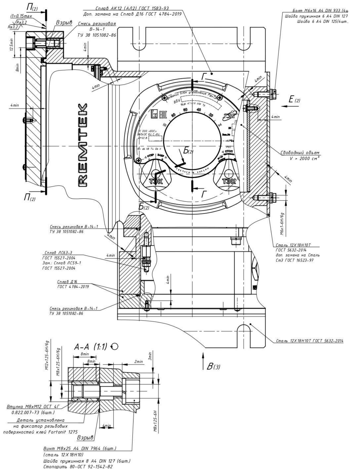
Рисунок И.1 – Чертеж взрывозащиты ВБУ (лист 1 из 6)
