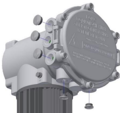
Рисунок 17 – Расположение транспортных заглушек
