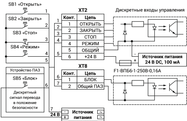
Пример подключения с использованием встроенного источника питания дискретных входов
