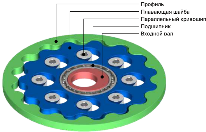
Циклоидальная передача
