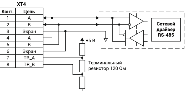
Структурная схема интерфейса RS-485
