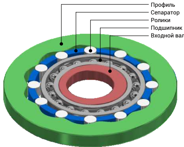
Волновая передача с промежуточными телами качения
