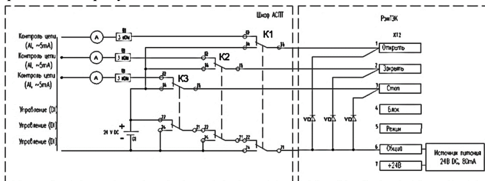
Рисунок 3 – Схема тестирования дискретных входов
