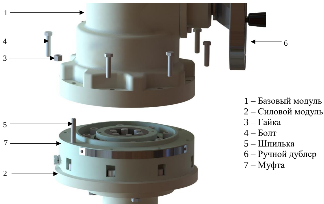
Рисунок 32 - Поворот БМ относительно редуктора
