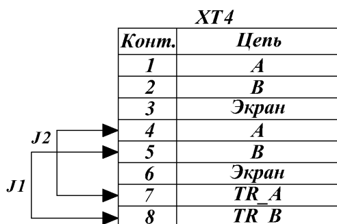
Рисунок 19 – Схема подключения с помощью перемычек
