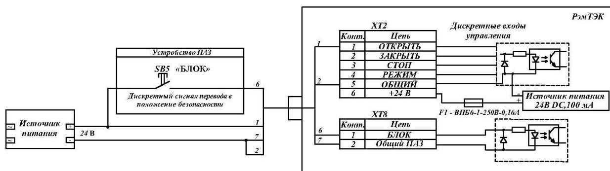
Рисунок 11 – Пример подключения электропривода для управления по двухпроводной однокомандной схеме управления
