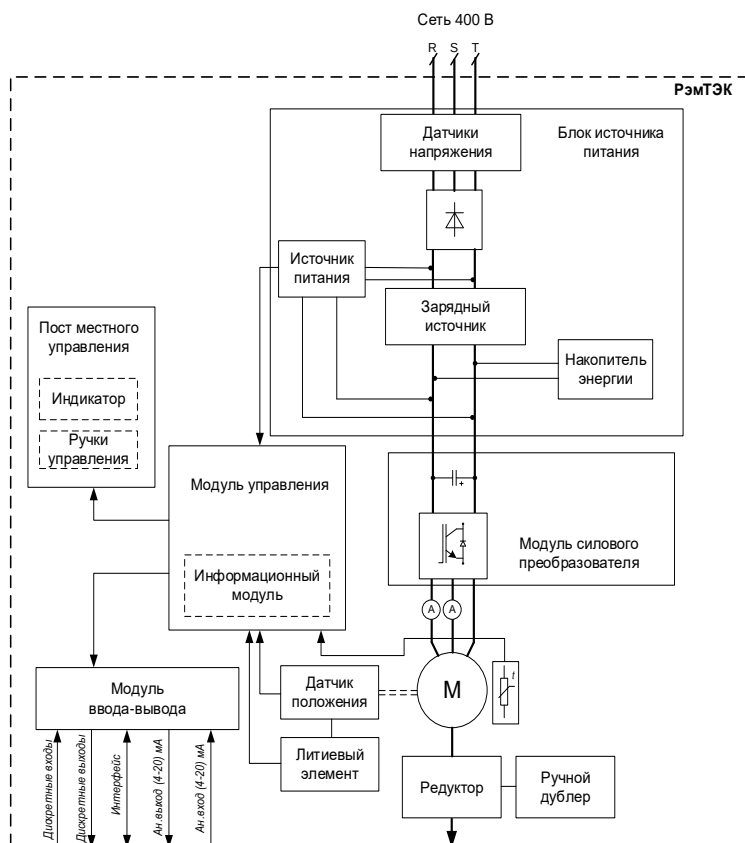
Рисунок 7 – Функциональная схема Базового модуля для электропривода «94» конструктивного исполнения
