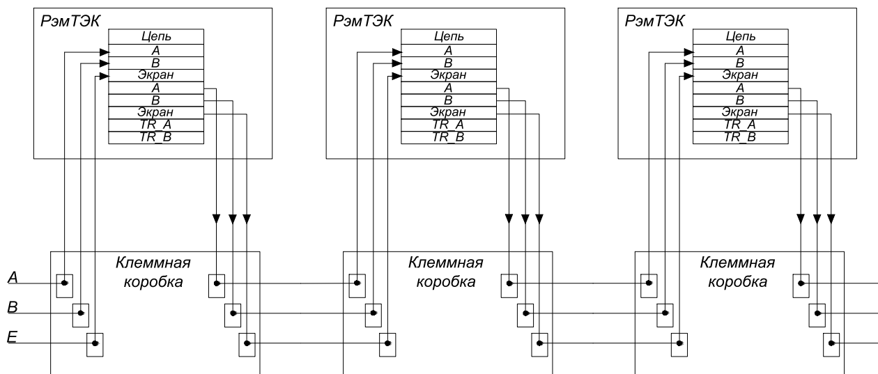
Рисунок 17 – Схема 1
