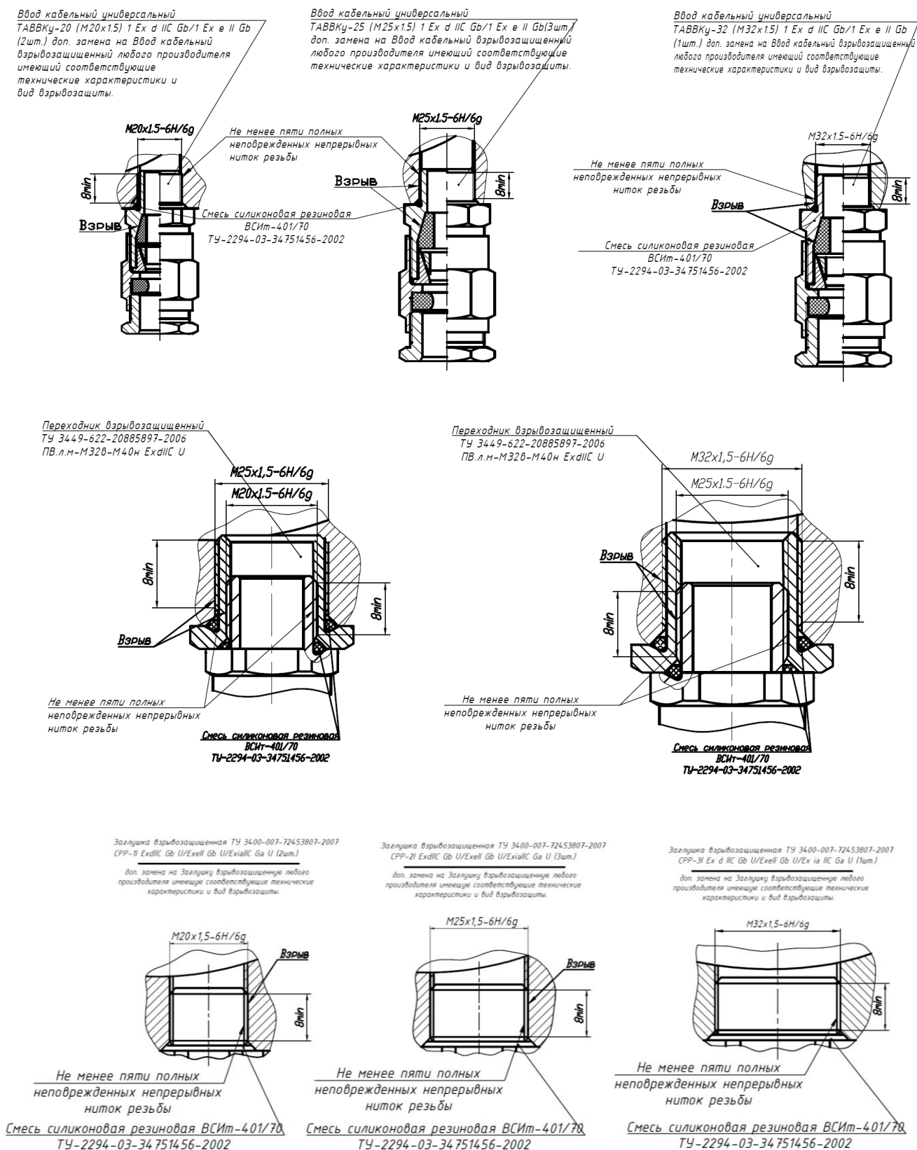
Рисунок Г.1 – Типы кабельных вводов, используемых в РэмТЭК
