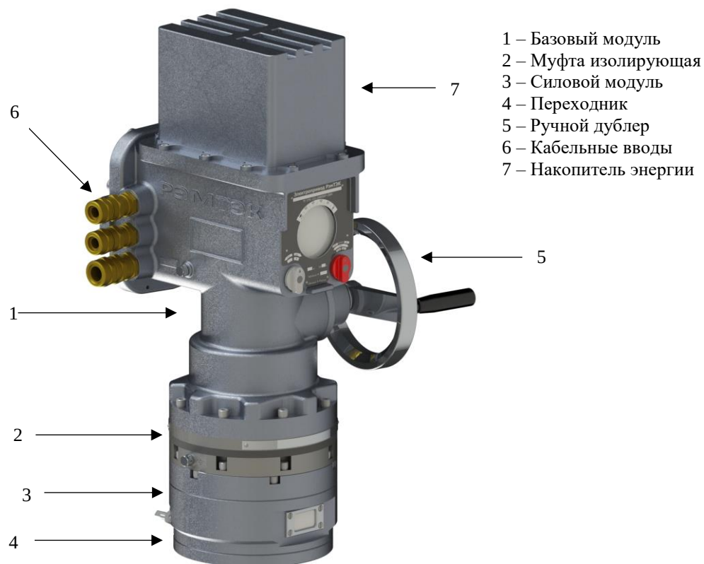
Рисунок 4 – Составные части электроприводов РэмТЭК конструктивного исполнения «91», «95»
