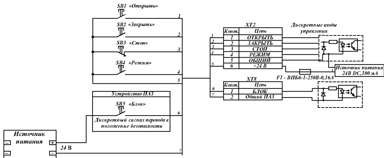
Рисунок 10 – Пример подключения с использованием встроенного источника питания дискретных входов
