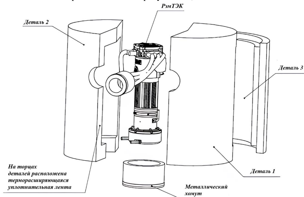
Рисунок 37 – Схема 1
