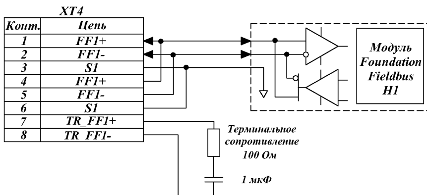
Рисунок 22 – Структурная схема подключения интерфейса Foundation Fieldbus
