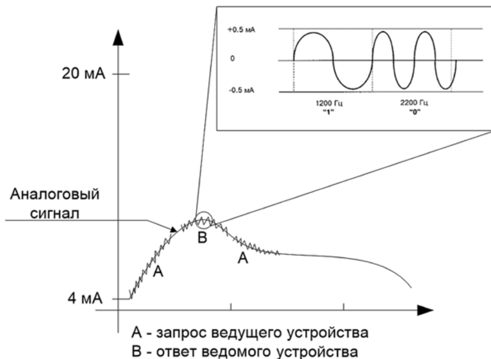
Рисунок 18 – Кодирование HART-сигнала
