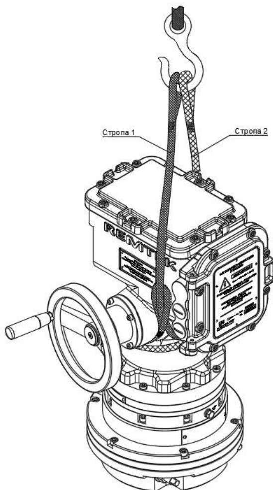
Рисунок 23 – Рекомендуемая схема строповки
