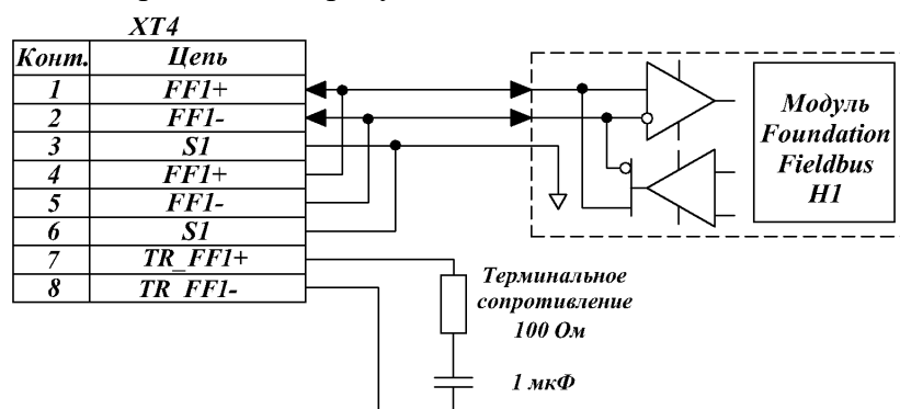
Рисунок 20 – Структурная схема подключения интерфейса Foundation Fieldbus
