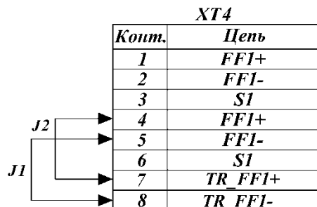
Рисунок 21 – Схема подключения терминального резистора на крайнем электроприводе
