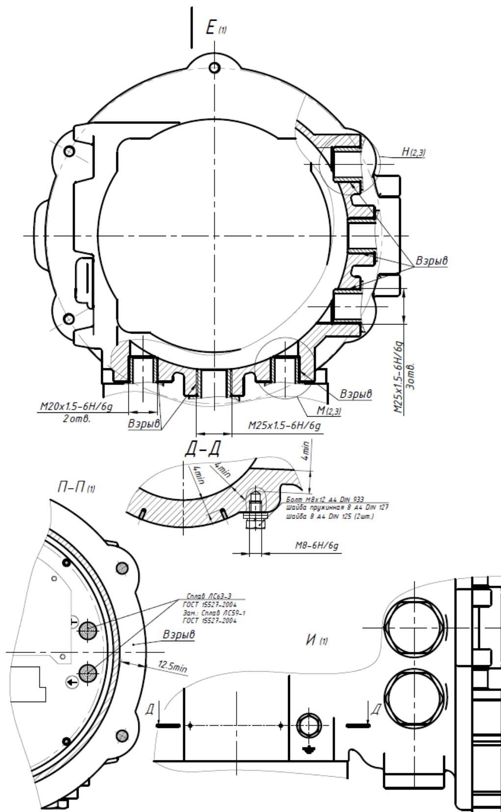
Рисунок Ж.2 – Чертеж средств взрывозащиты базового модуля БМ.87.х.х.хх.02.хх.ххххх (лист 3 из 9)
