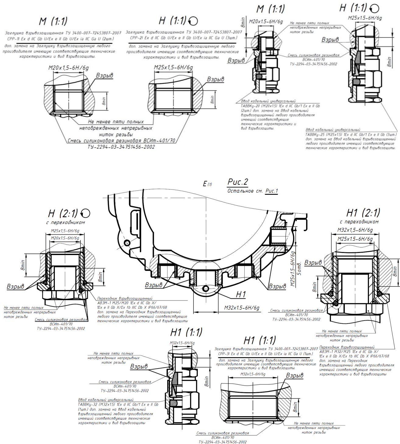
Рисунок Ж.2 – Чертеж средств взрывозащиты базового модуля БМ.87.х.х.хх.02.хх.хххх (лист 4 из 9)
