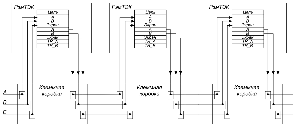
Рисунок 15 – Рекомендованное соединение электроприводов при использовании клеммной коробки
