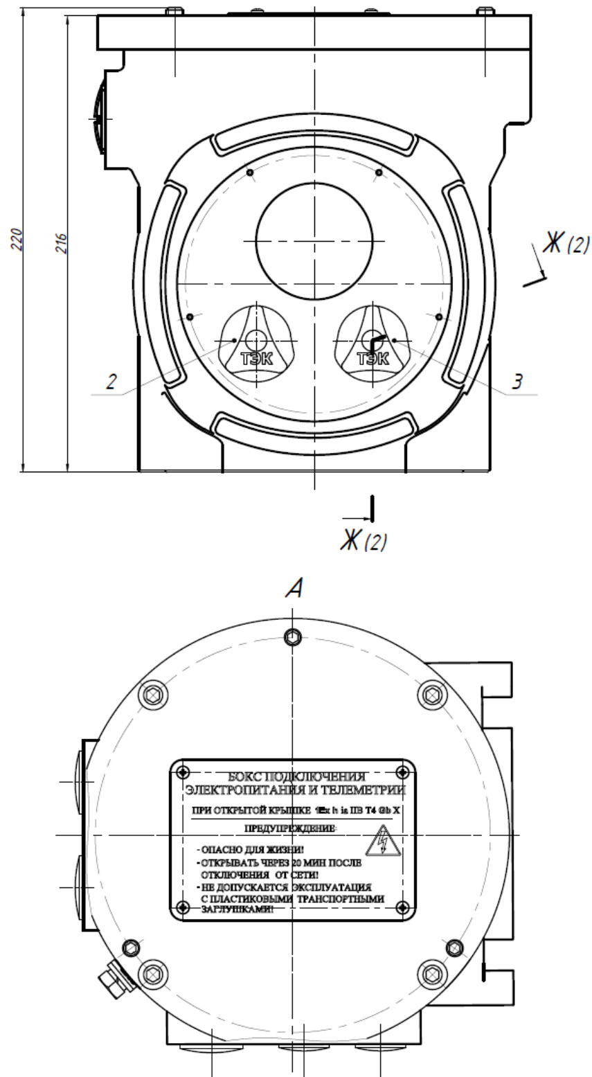
Рисунок Ж.3 – Чертеж средств взрывозащиты базового модуля БМ.86.x.x.xx.01.xx.xxxx (лист 7 из 13)
