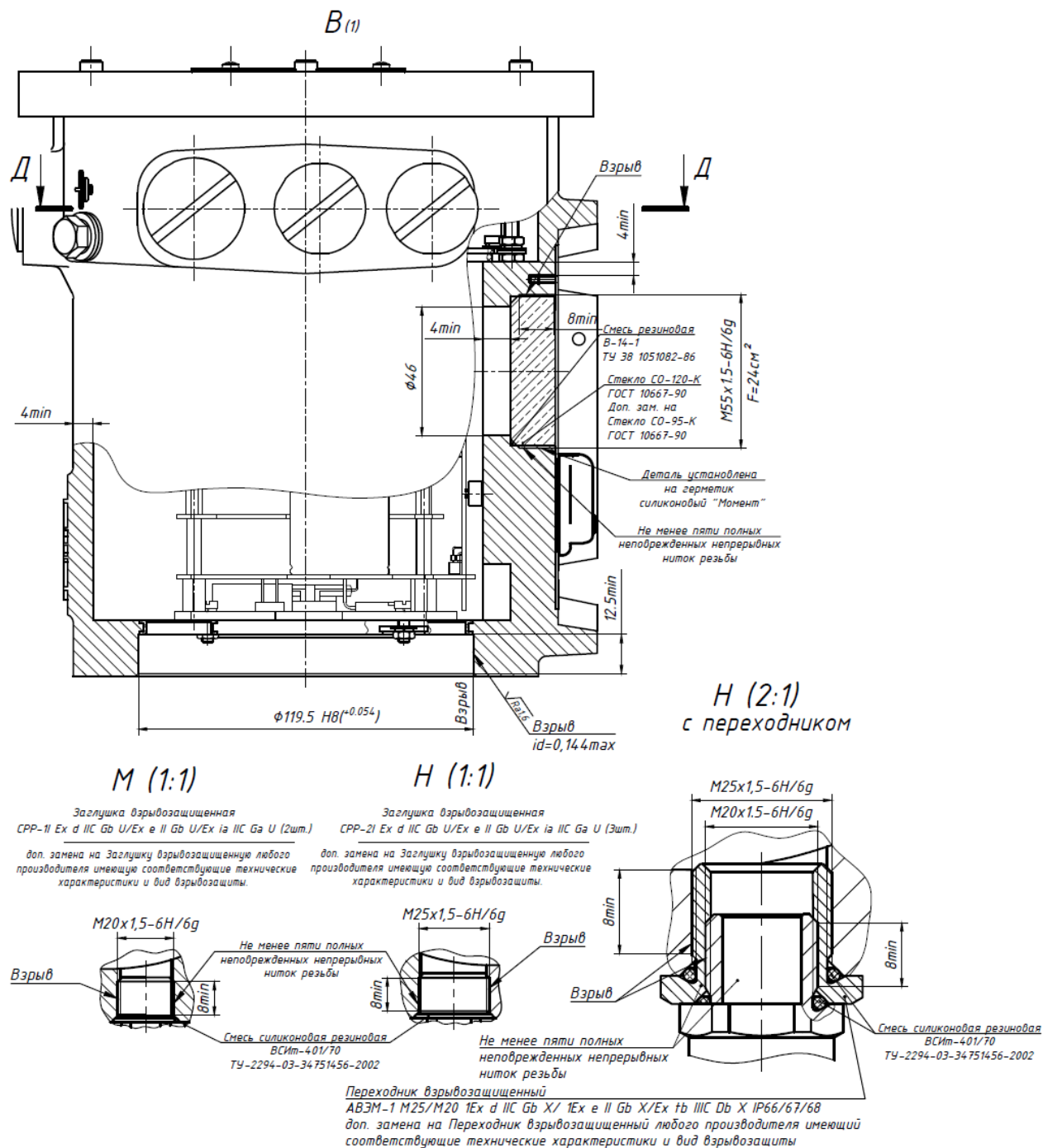
Рисунок Ж.3 – Чертеж средств взрывозащиты базового модуля БМ.86.x.x.xx.01.xx.xxxx (лист 3 из 13)
