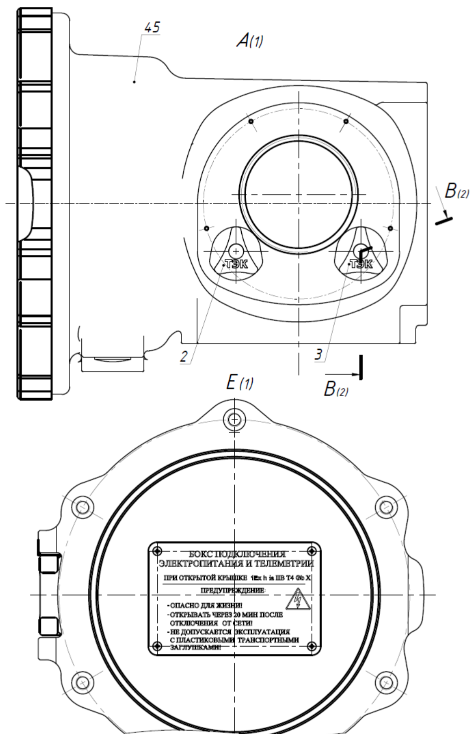
Рисунок Ж.2 – Чертеж средств взрывозащиты базового модуля БМ.87.x.x.xx.02.xx.xxxx (лист 5 из 9)
