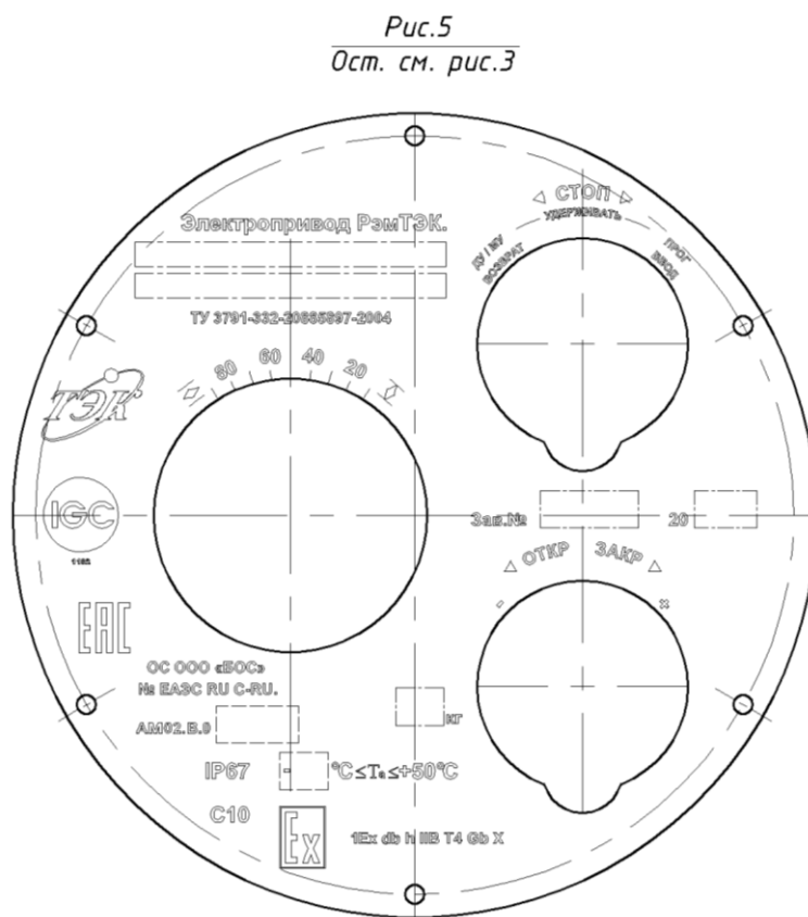
Рисунок Ж.3 – Чертеж средств взрывозащиты базового модуля БМ.86.х.х.хх.01.хх.хххх (лист 11 из 13)
