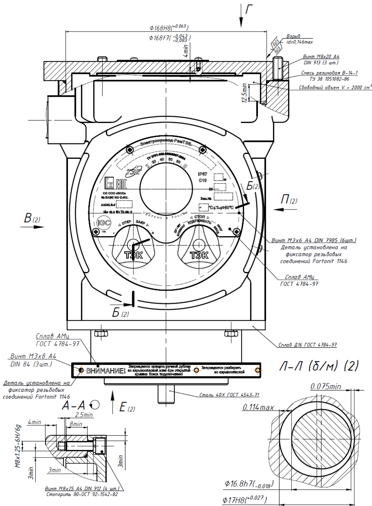
Рисунок Ж.4 – Чертеж средств взрывозащиты базового модуля БМ.83.V.2.xx.xx.xx.UXII1 (лист 1 из 9)
