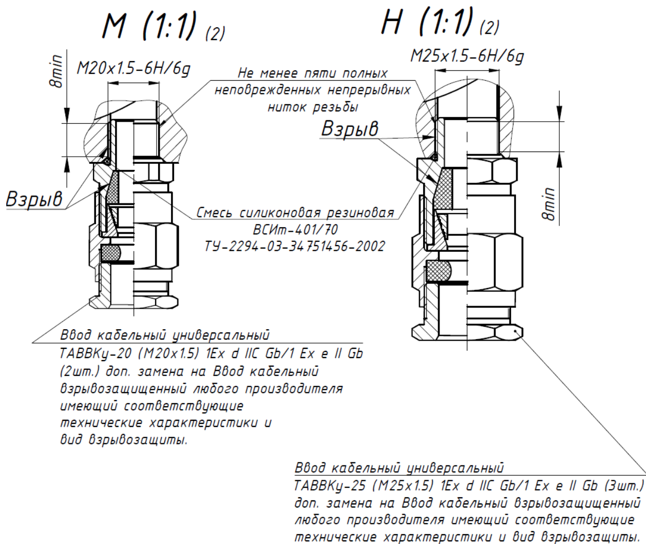
Рисунок Ж.4 – Чертеж средств взрывозащиты базового модуля БМ.83.V.2.xx.xx.xx.УХЛ1 (лист 3 из 9)
