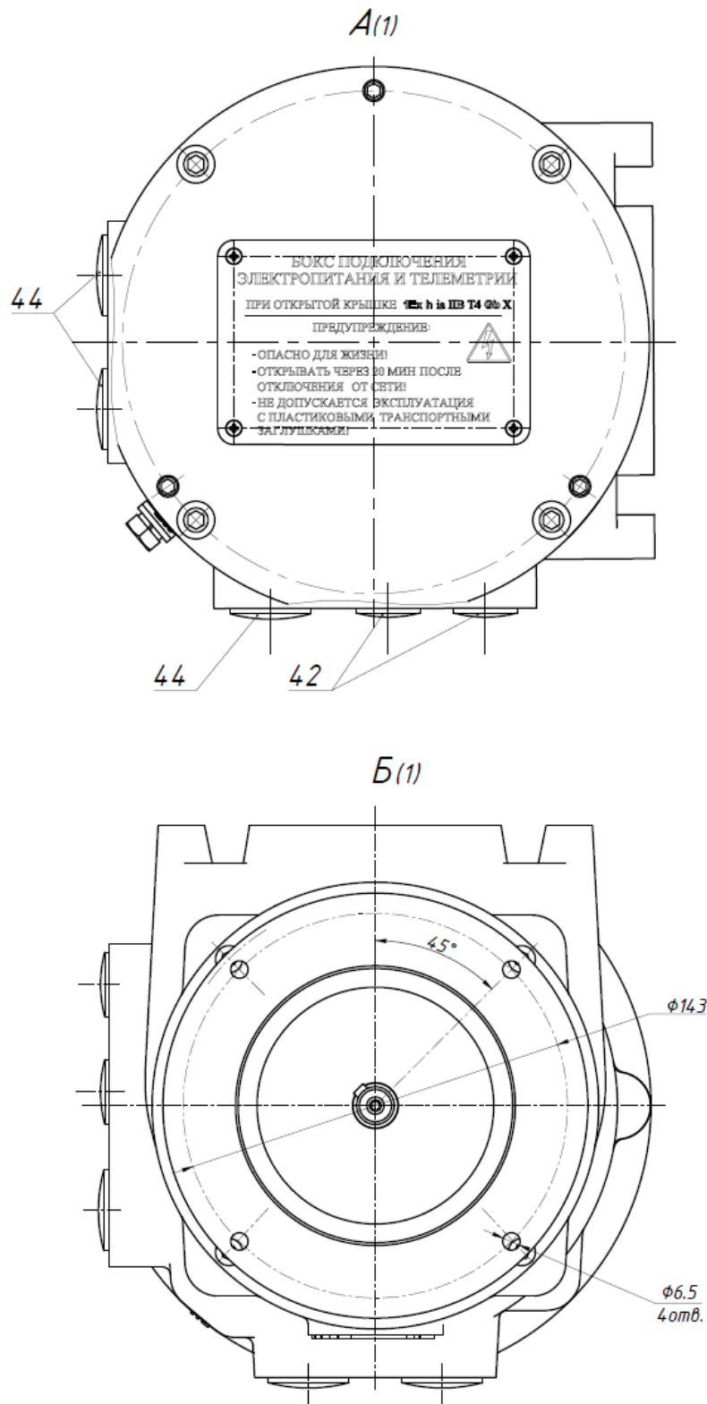
Рисунок Ж.4 – Чертеж средств взрывозащиты базового модуля БМ.83.V.2.xx.xx.xx.UXL1 (лист 7 из 9)
