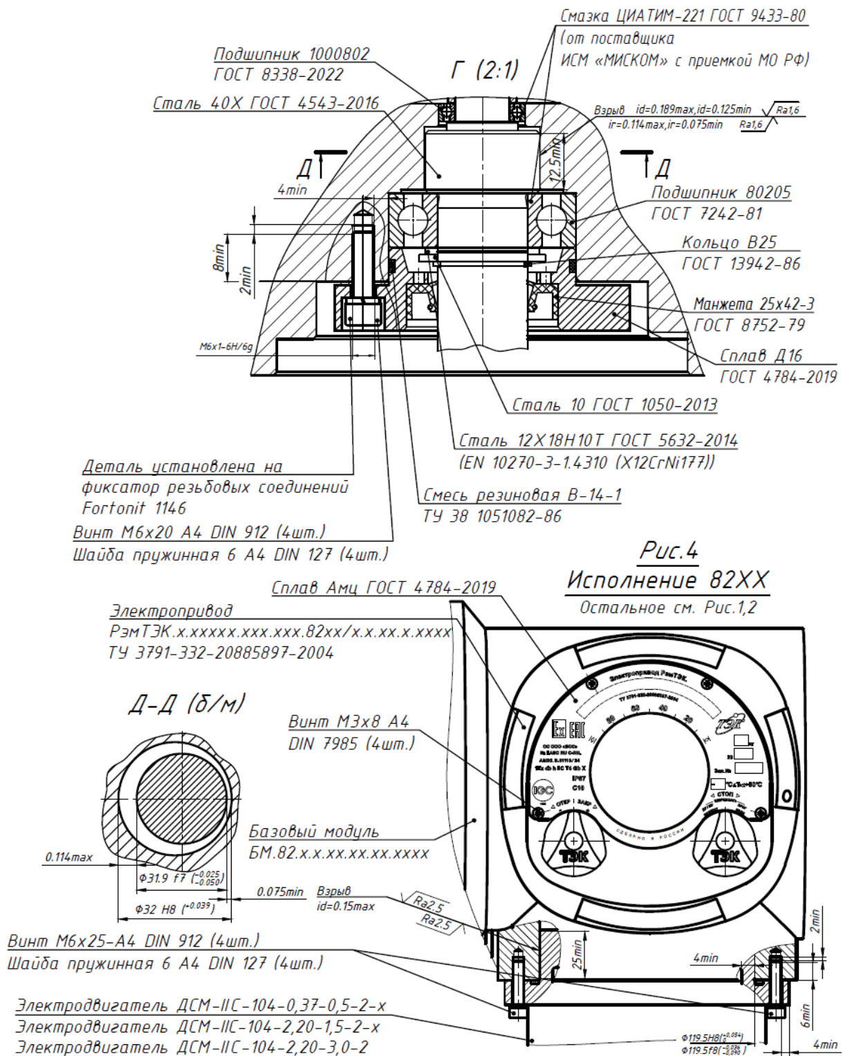
Рисунок Ж.1 – Чертеж средств взрывозащиты РэмТЭК.Л.ххххх.ххх.ххх.хххх/х.х.хх.х.УХЛ1 (лист 4 из 4)
