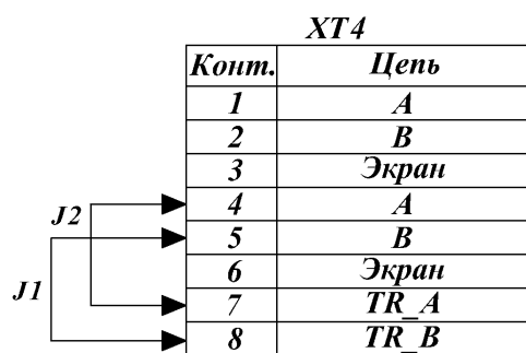
Рисунок 17 – Структурная схема подключения с помощью перемычек
