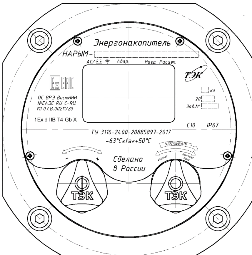
Рисунок 2 – Внешний вид ПМУ энергонакопителя
