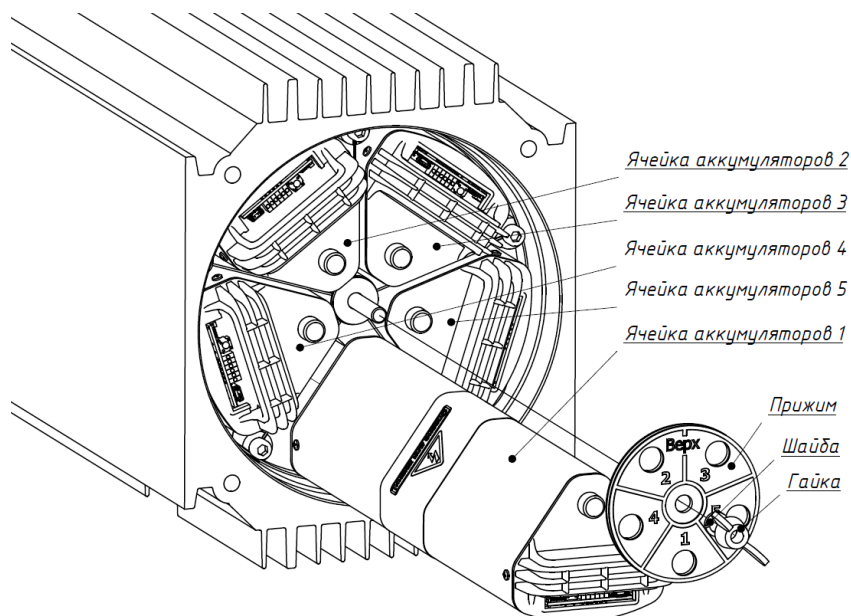
Рисунок 5 – Замена аккумуляторов в энергонакопителе 1125 кДж
