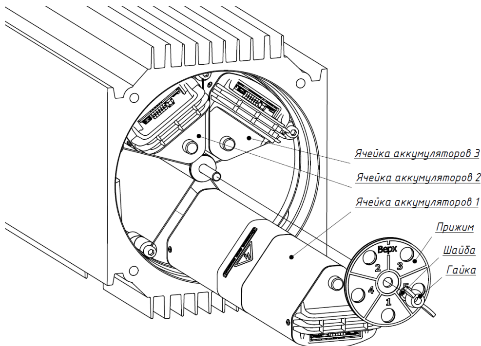
Рисунок 6 – Замена аккумуляторов в энергонакопителе 675 кДж
