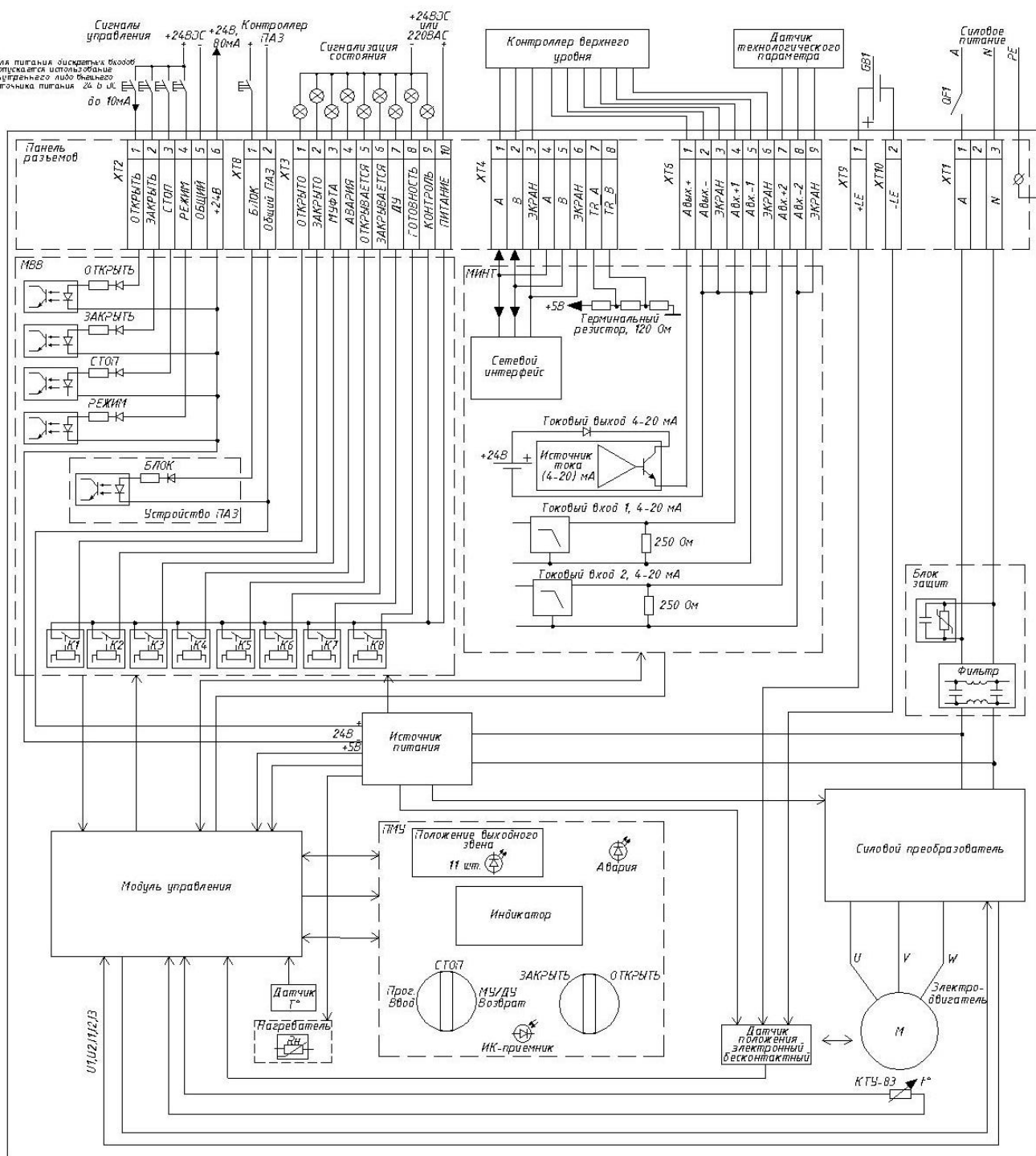
Рисунок Ж.1 – Схема электрическая функциональная РэмТЭК при питании от однофазной цепи переменного тока напряжением 230 В частотой 50 Гц
