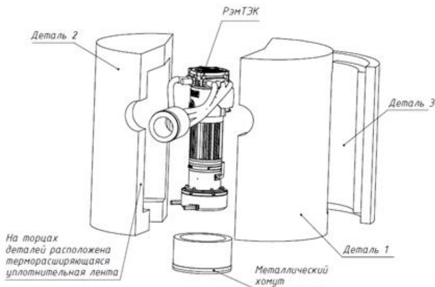
Рисунок 37 – Схема 1
