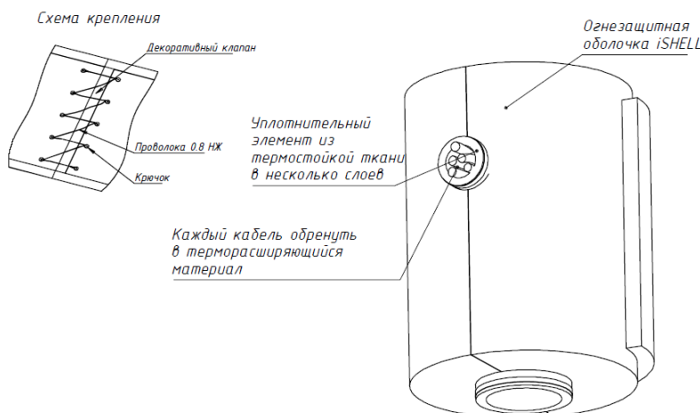
Рисунок 38 – Схема 2
