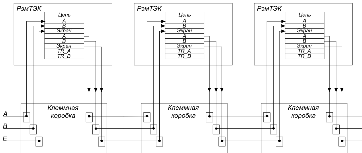
Рисунок 17 – Схема 1
