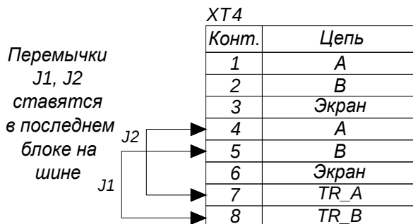
Рисунок 19 – Схема подключения с помощью перемычек
