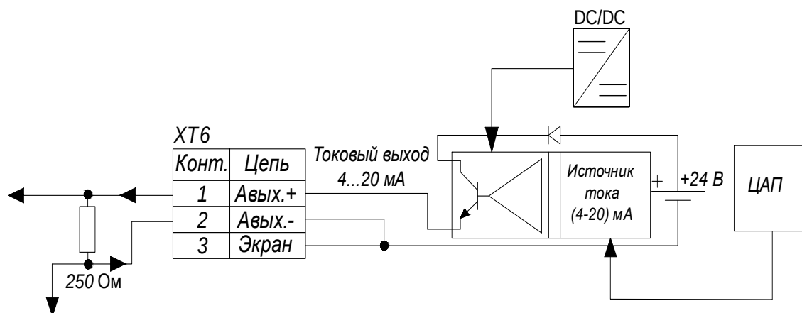
Рисунок 15 – Структурная схема аналогового выхода
