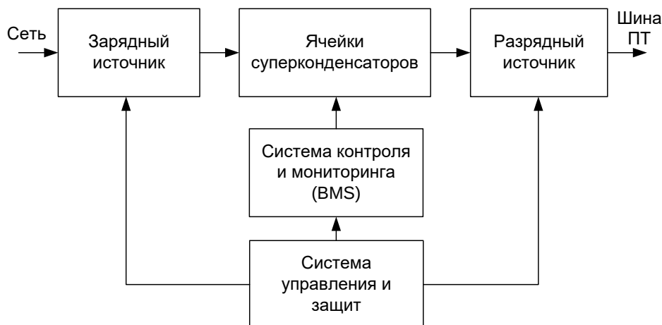
Рисунок 24 – Структурная схема энергоаккумулятора для РэмТЭК «91», «95» конструктивного исполнения
