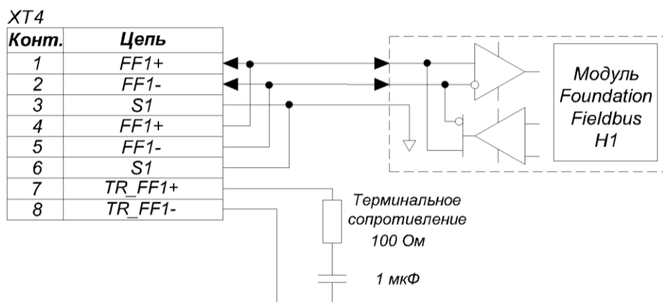
Рисунок 22 – Структурная схема подключения интерфейса Foundation Fieldbus
