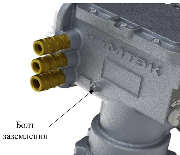
Рисунок 33 - Заземление электропривода
