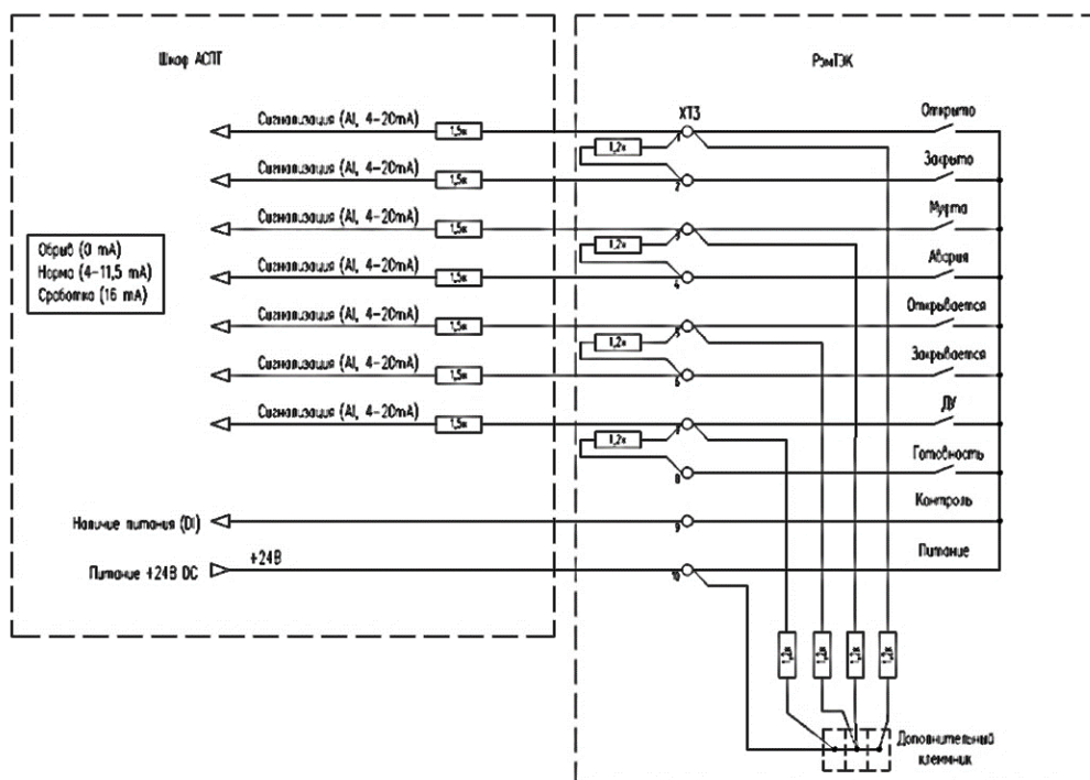
Рисунок 13 – Схема диагностики состояния дискретных выходов РэмТЭК
