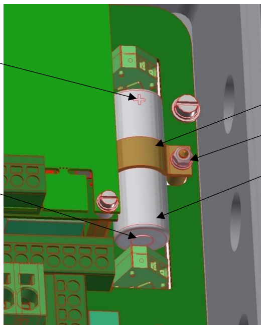
Рисунок 44 – Замена литиевого элемента
