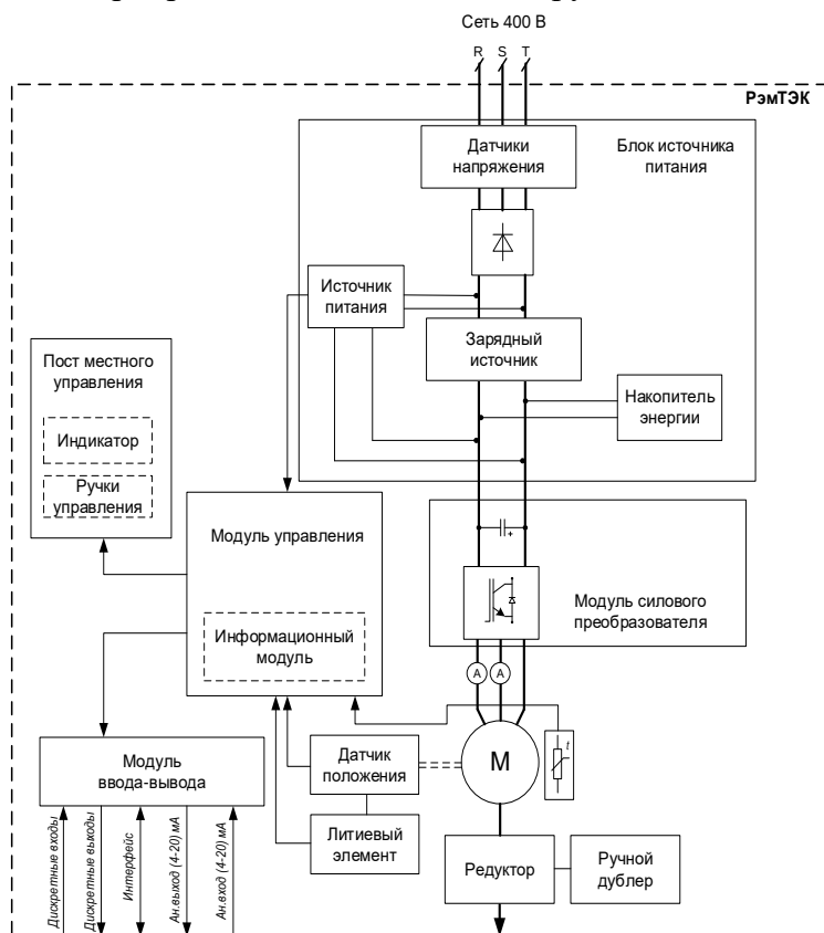
Рисунок 6 – Функциональная схема Базового модуля для электроприводов «91», «95» конструктивного исполнения
