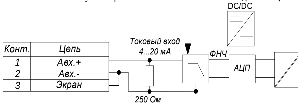
Рисунок 14 – Структурная схема аналогового входа
