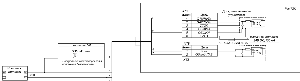
Рисунок 11 – Пример подключения электропривода для управления по двухпроводной однокомандной схеме управления
