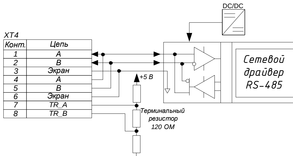
Рисунок 16 – Структурная схема интерфейса RS-485
