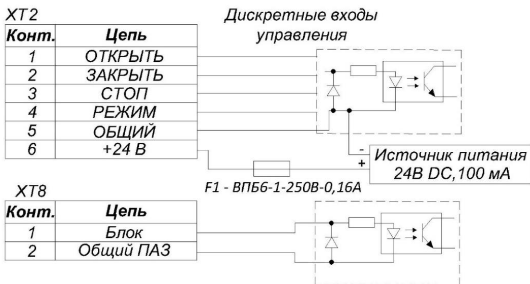
Рисунок 9 – Структурная схема дискретного входа
