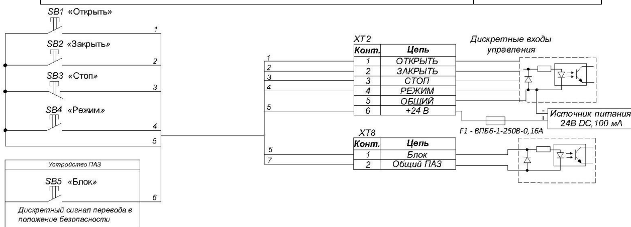
Рисунок 10 – Пример подключения с использованием встроенного источника питания дискретных входов
