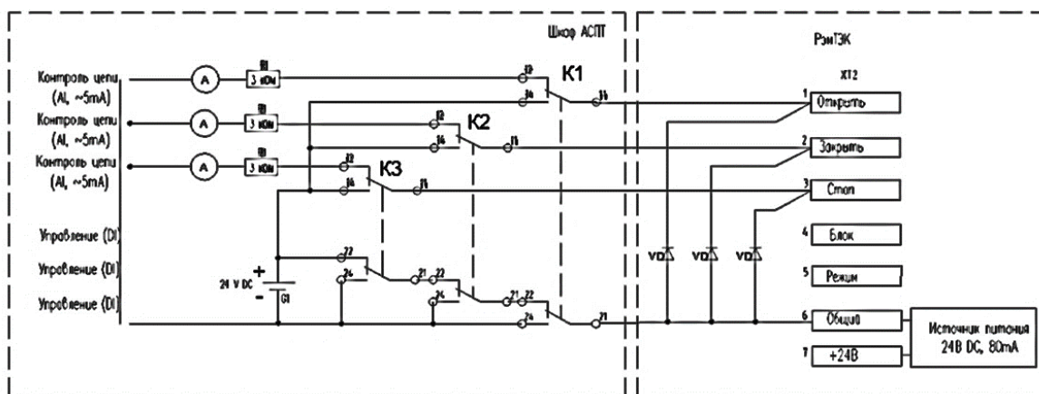
Рисунок 12 – Схема тестирования дискретных входов
