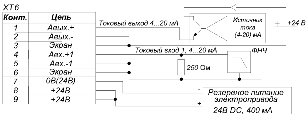
Рисунок 27 – Схема подключения
