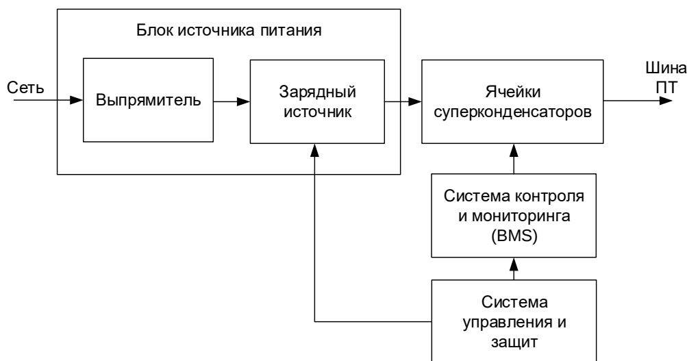
Рисунок 25 – Структурная схема энергоаккумулятора для РэмТЭК «94» конструктивного исполнения
