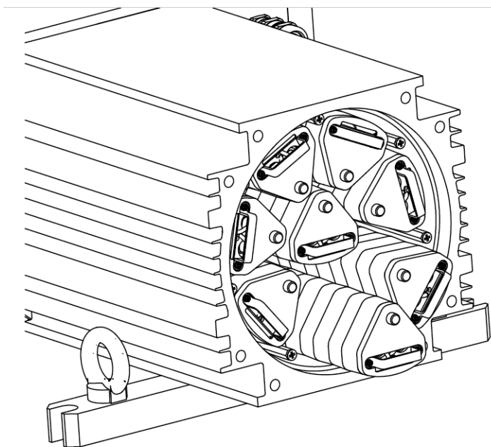
Рисунок 6 – Замена аккумуляторов в энергонакопителе НАРЫМ-3375
