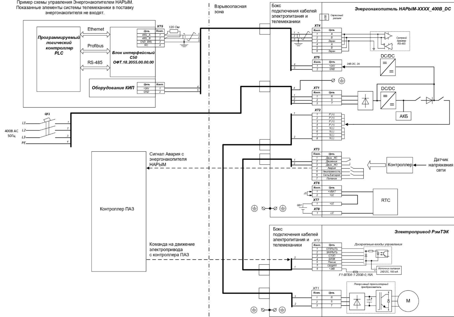
Рисунок Г.1 – Схема подключения энергонакопителя при трехфазном напряжении питания 400 В
