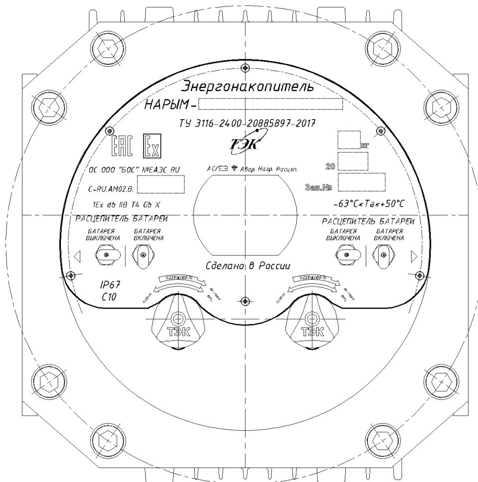
Рисунок 2 – Внешний вид ПМУ энергонакопителя
