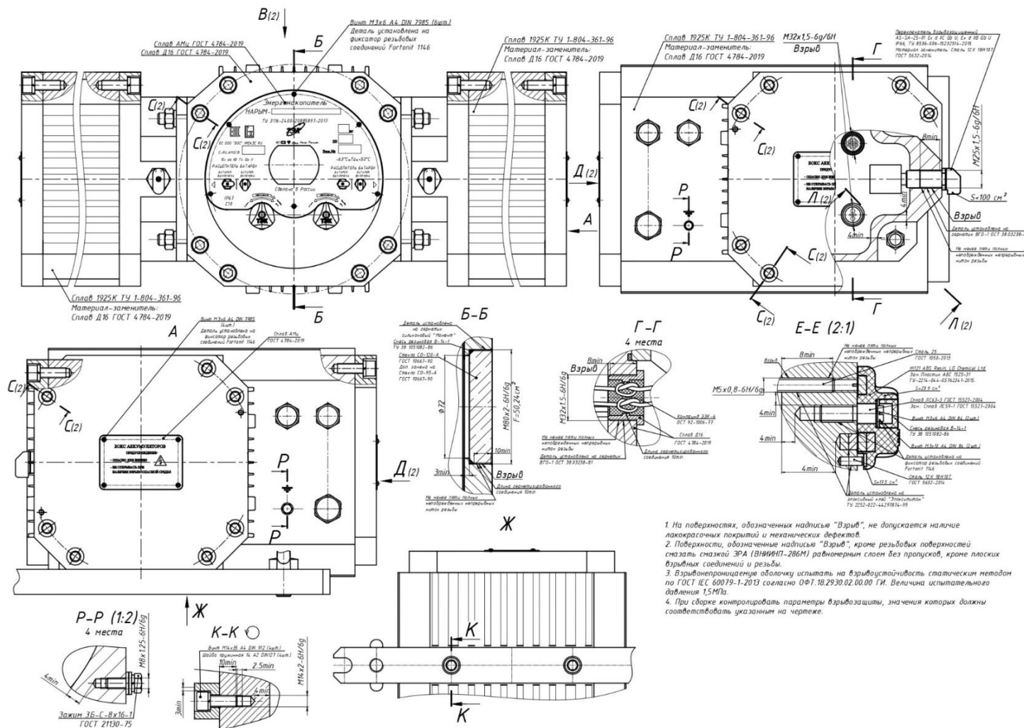
Рисунок В.1 – Чертеж средств взрывозащиты
