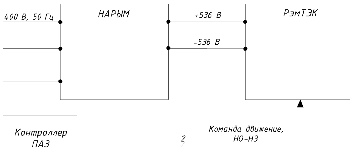
Рисунок 4 - Схема подключения с формированием сигнала команды с контроллера ПАЗ
