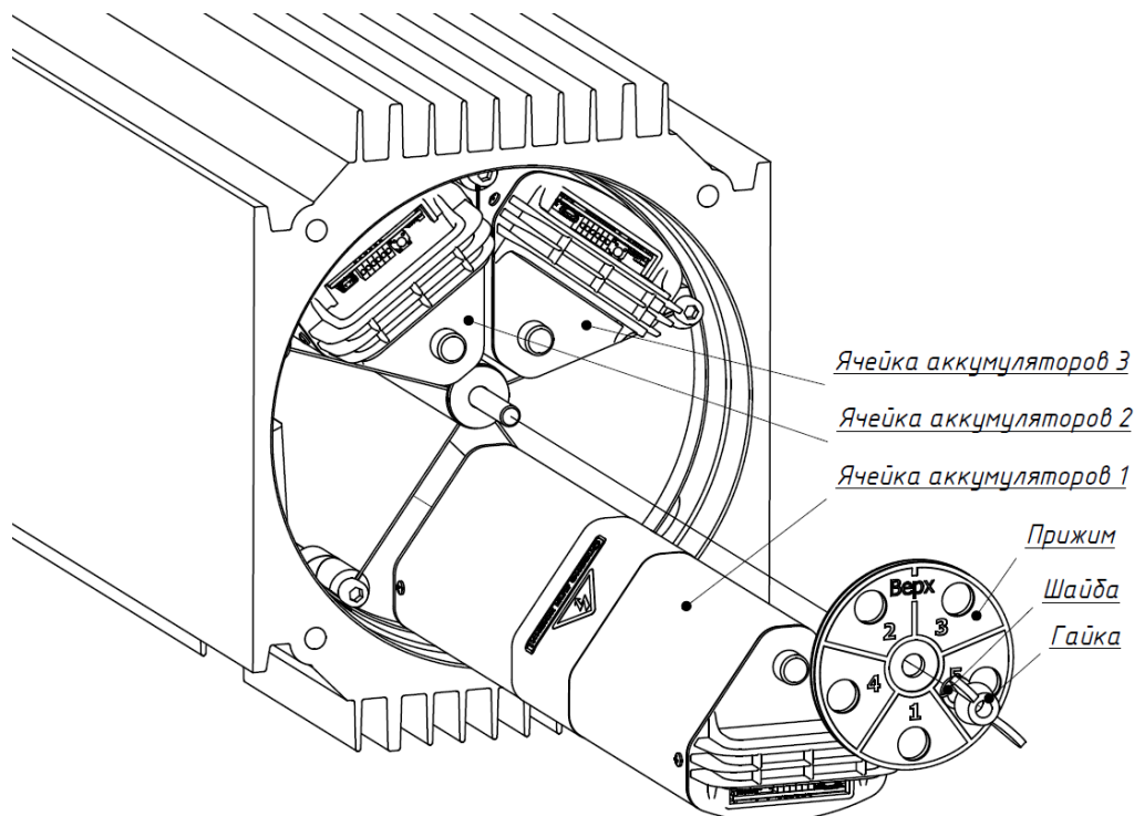
Рисунок 6 – Замена аккумуляторов в энергонакопителе 675 кДж
