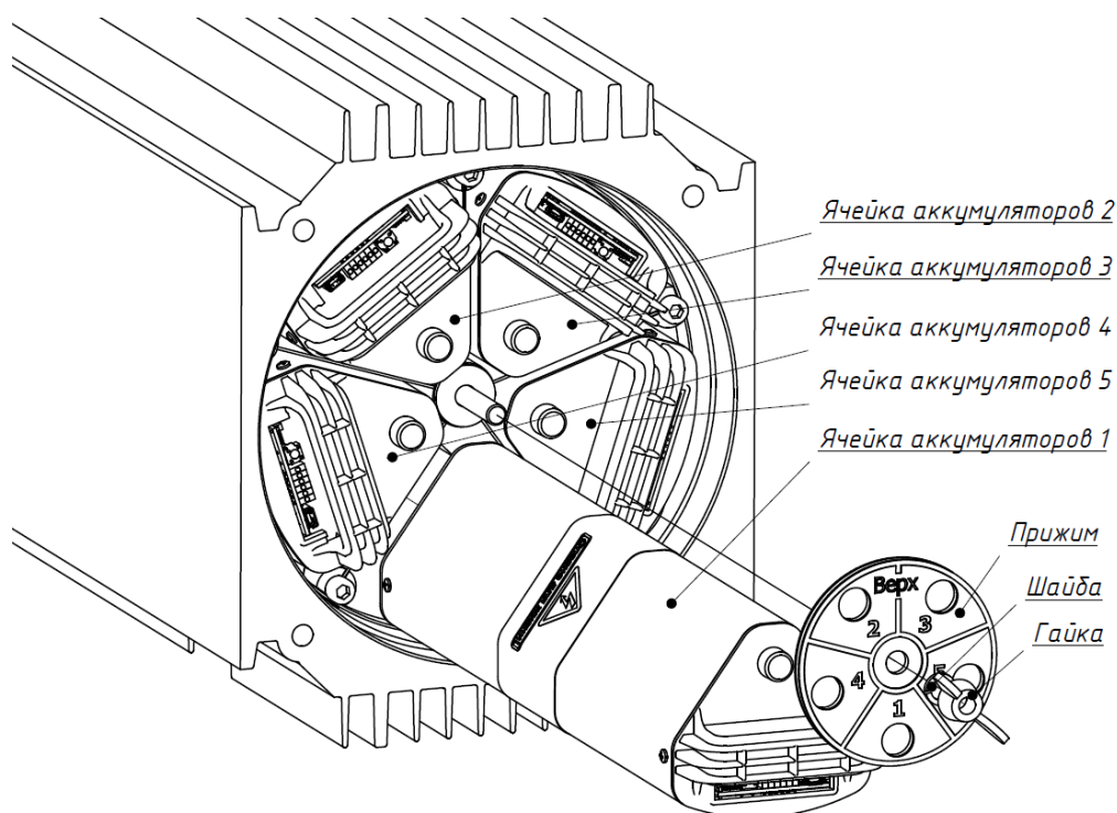
Рисунок 5 – Замена аккумуляторов в энергонакопителе 1125 кДж
