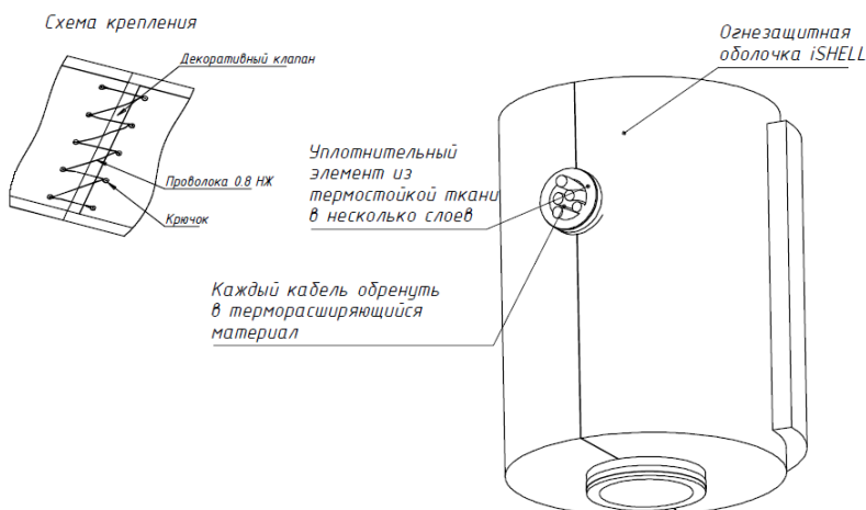
Рисунок 18г – Монтаж термочехла
