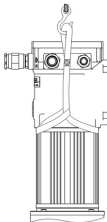
Рисунок 13 – Рекомендуемая схема строповки РэмТЭК без рым-болтов
