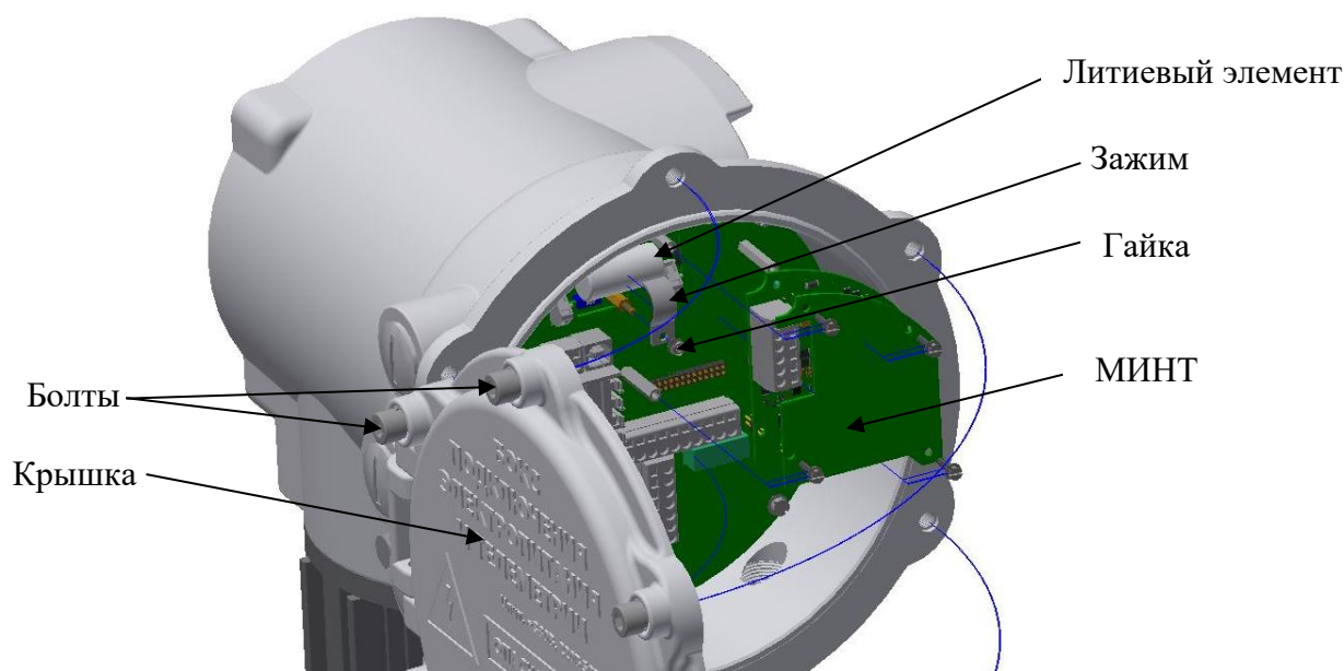
Рисунок 22 – Замена литиевого элемента РэмТЭК
