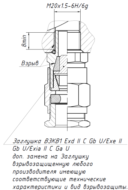
Рисунок 186 – Способ установки взрывозащищенной пробки в кабельный ввод
