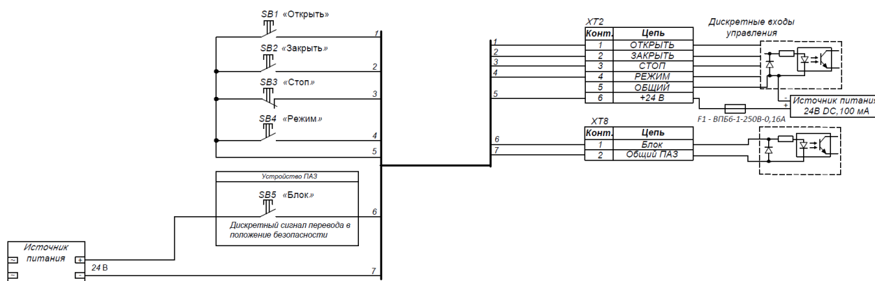
Рисунок 8 – Пример подключения с использованием встроенного источника питания дискретных входов
