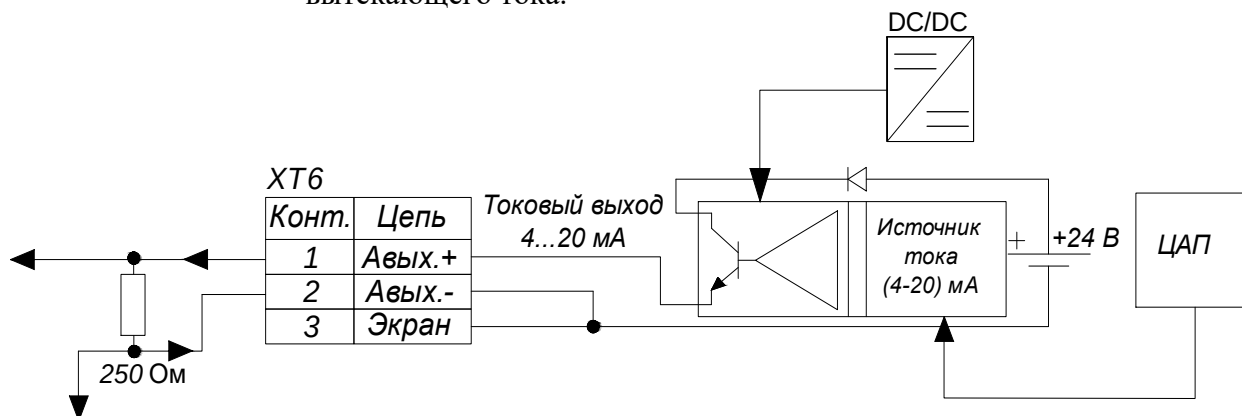
Рисунок 11 – Структурная схема аналогового выхода
