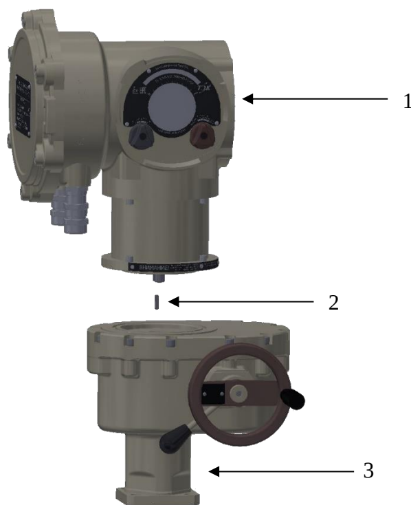
Рисунок 24 – Порядок замены редуктора
