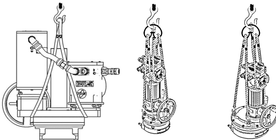
Рисунок 13а – Рекомендуемые схемы строповки РэмТЭК с рым-болтами
