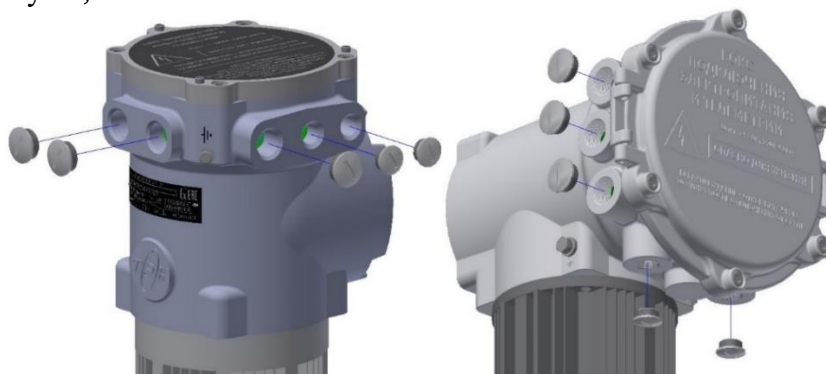
Рисунок 17 – Расположение транспортных заглушек
