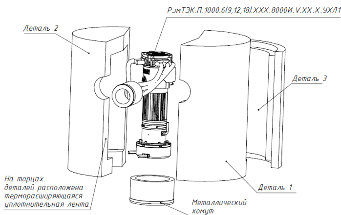
Рисунок 18в – Монтаж термочехла
