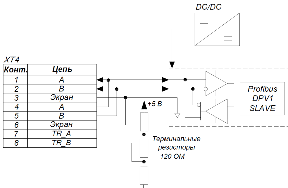
Рисунок 12ж – Структурная схема интерфейса Profibus DP
