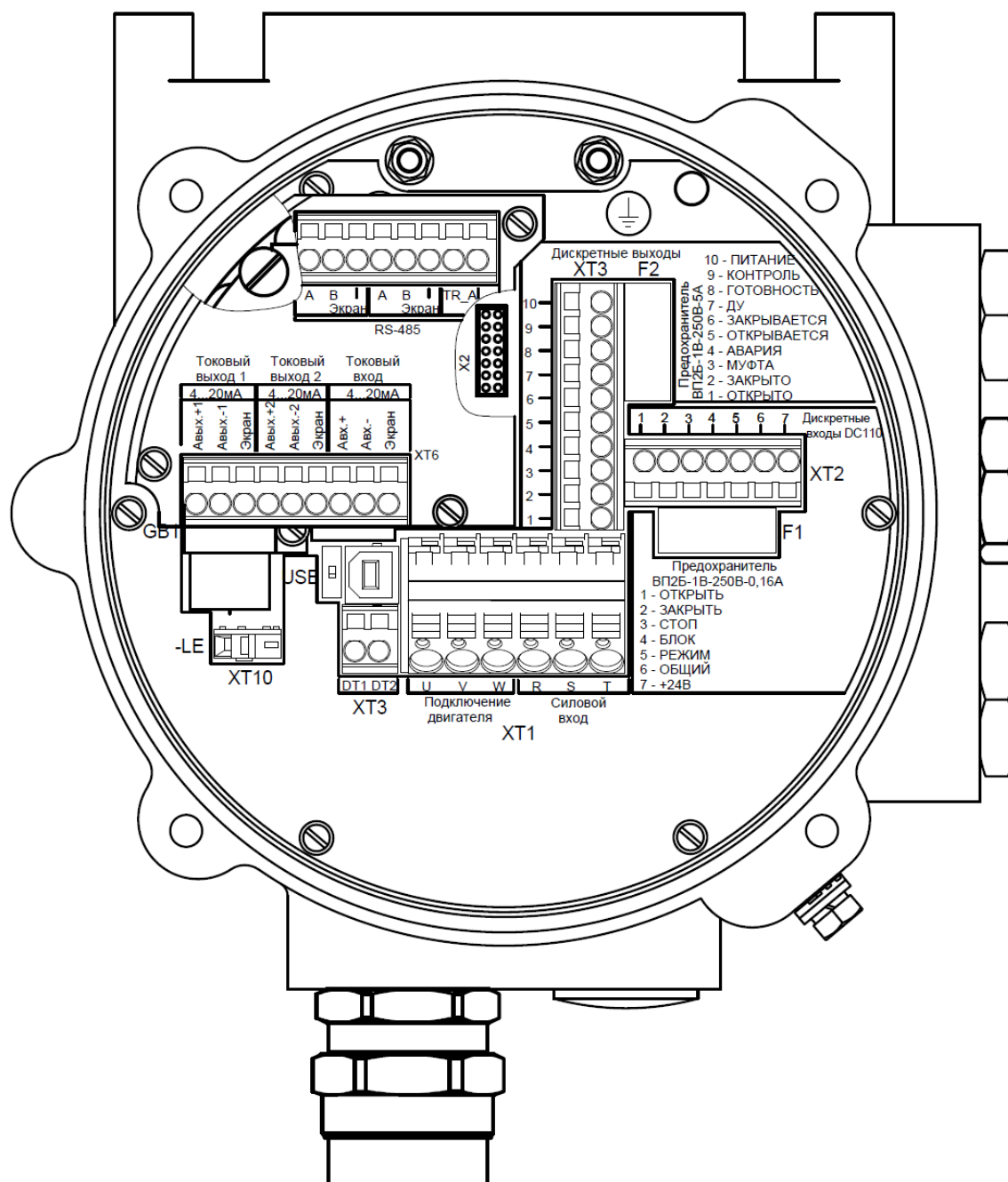
Рисунок 18 – Типовой внешний вид бокса РэмТЭК конструктивного исполнения «8xxx»
