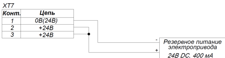
Рисунок 12и – Схема резервного питания электропривода для модификаций «17», «18», «19», «45»
