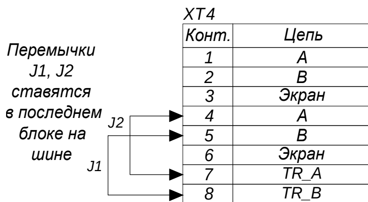
Рисунок 12г – Структурная схема подключения с помощью перемычек
