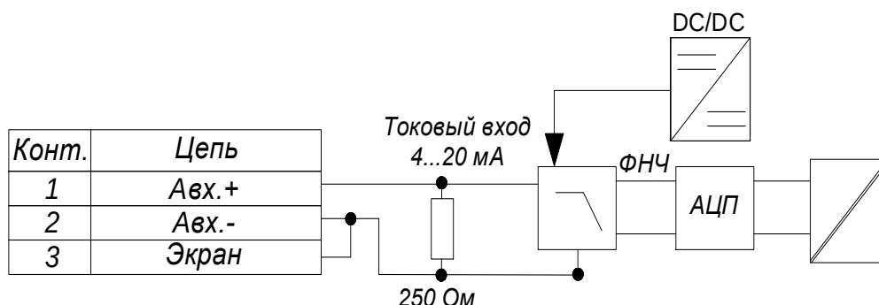
Рисунок 10а – Структурная схема аналогового входа
