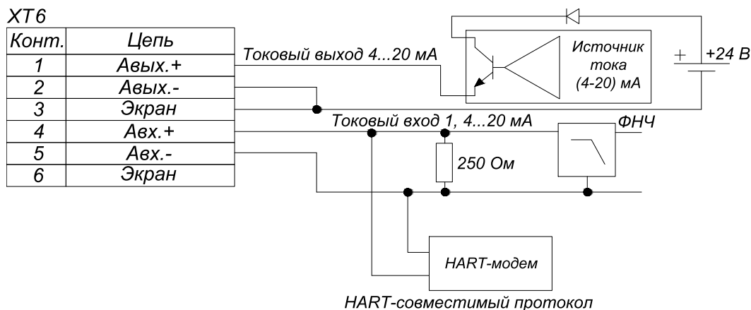
Рисунок 12е – Структурная схема HART-интерфейса
