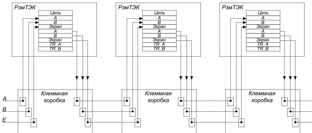
Рисунок 126 – Рекомендованное соединение электроприводов при использовании клеммной коробки
