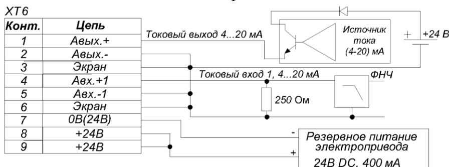
Рисунок 12и – Схема резервного питания электропривода для модификаций «17», «18», «19», «45»
