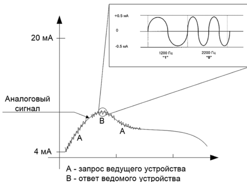
Рисунок 12д – Кодирование HART-сигнала
