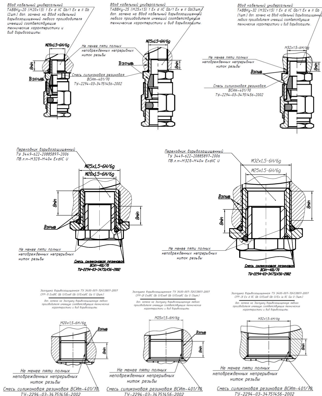
Рисунок В.1 – Типы кабельных вводов, используемых в РЭМТЭК
