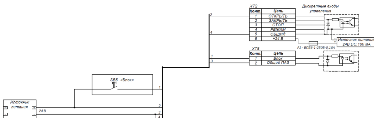
Рисунок 9 – Пример подключения электропривода для управления по двухпроводной однокомандной схеме управления
