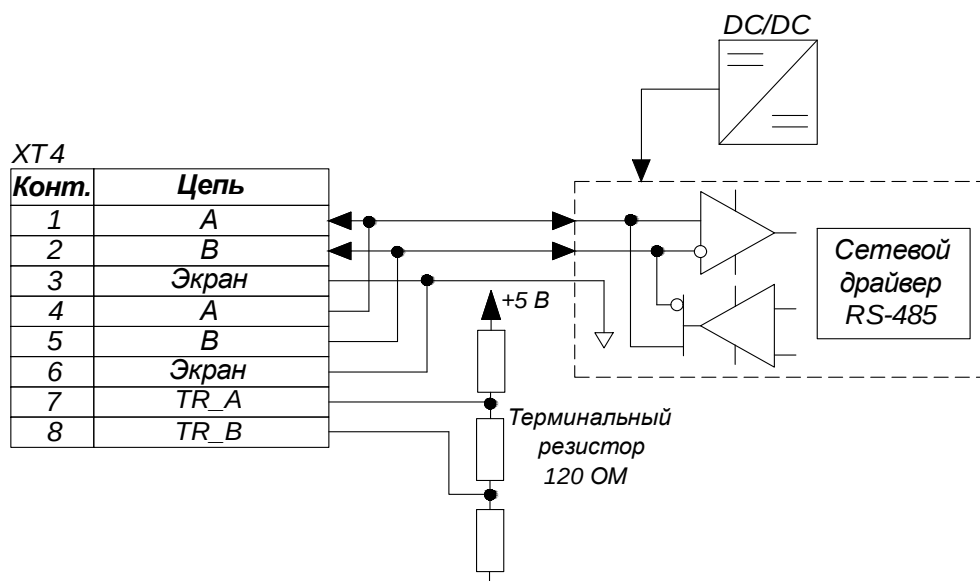
Рисунок 12а – Структурная схема интерфейса RS-485
