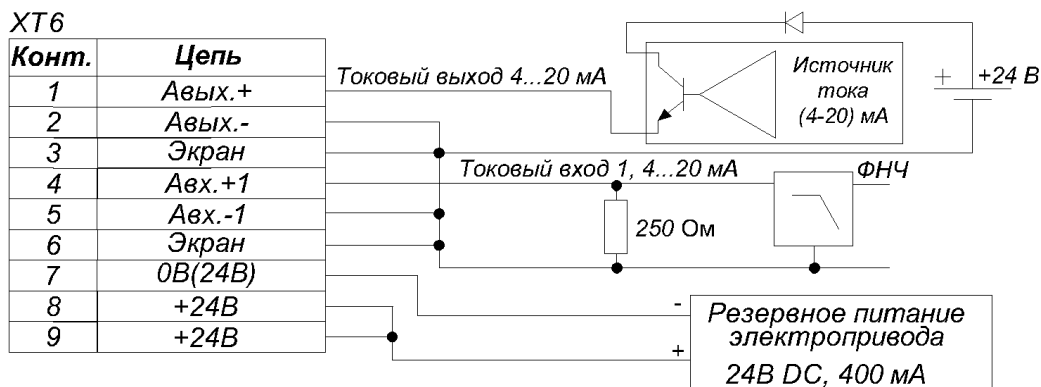
Рисунок 27 – Схема подключения
