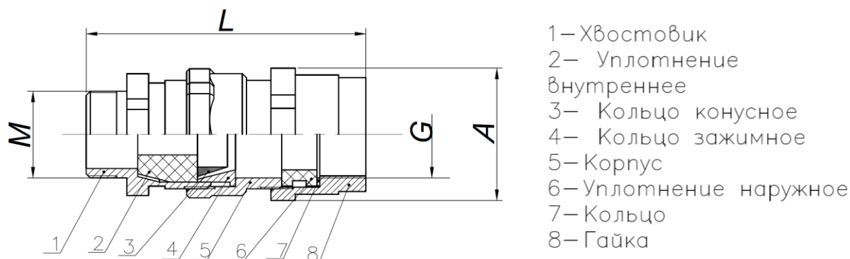
Рисунок Е.1 – Кабельный ввод ТАВВКу
