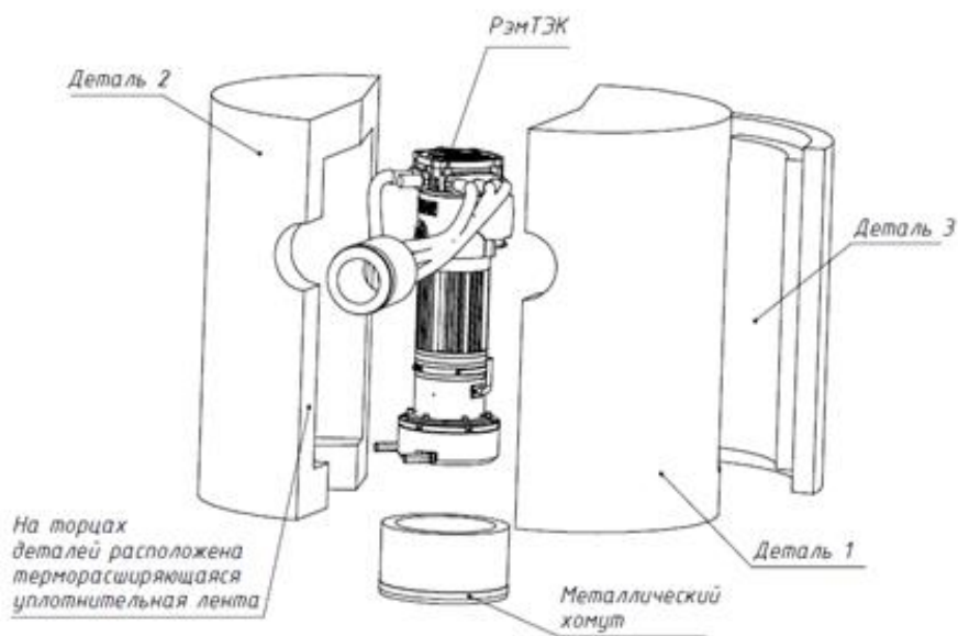
Рисунок 31 – Схема 1
