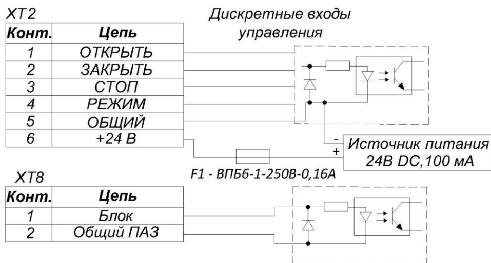
Рисунок 7 - Структурная схема дискретного входа
