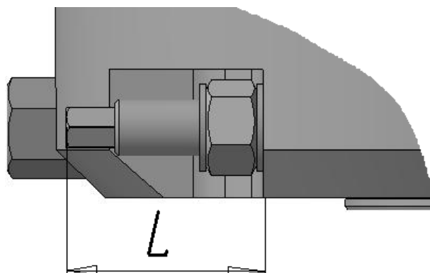
Рисунок 33 - Заглушка снята
