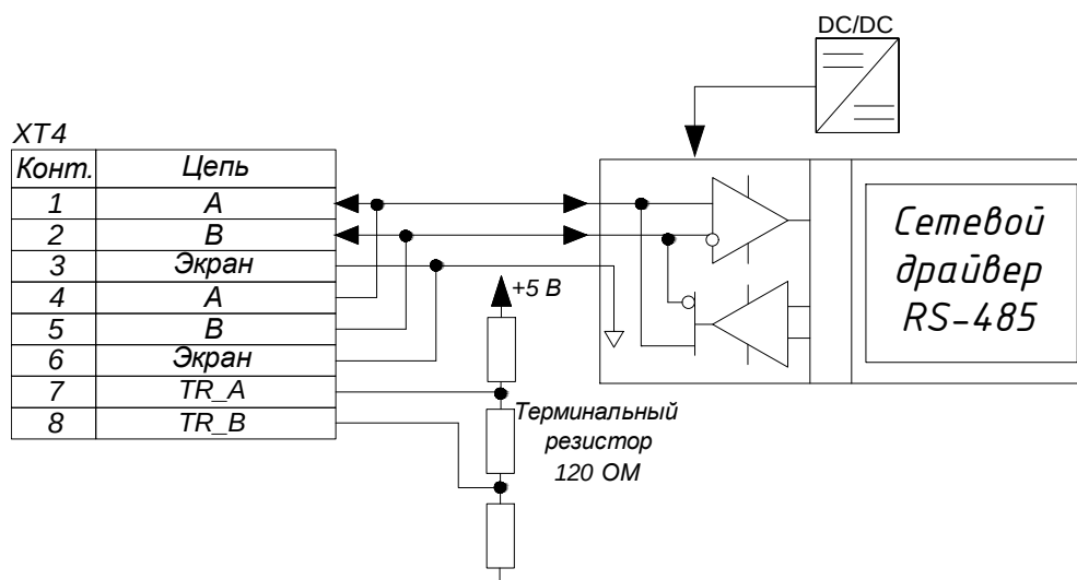
Рисунок 14 – Структурная схема RS-485
