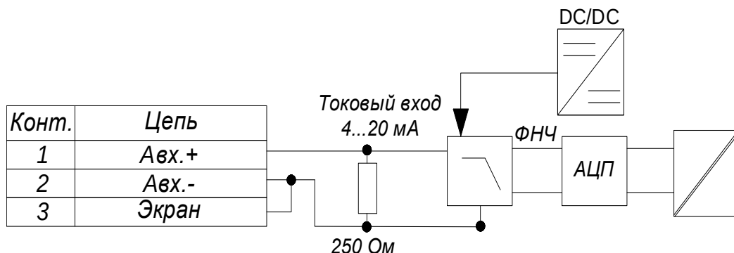
Рисунок 12 – Структурная схема аналогового входа
