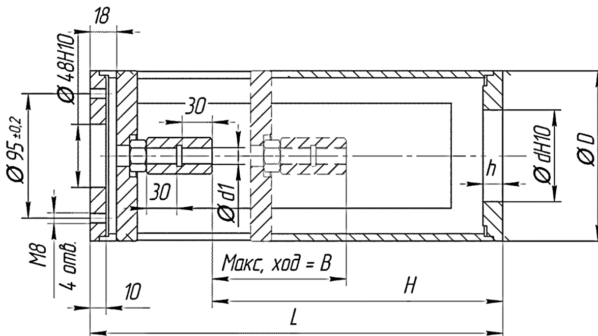
Рисунок Г.3 – Присоединительное звено прямоходных РэмТЭК к арматуре
