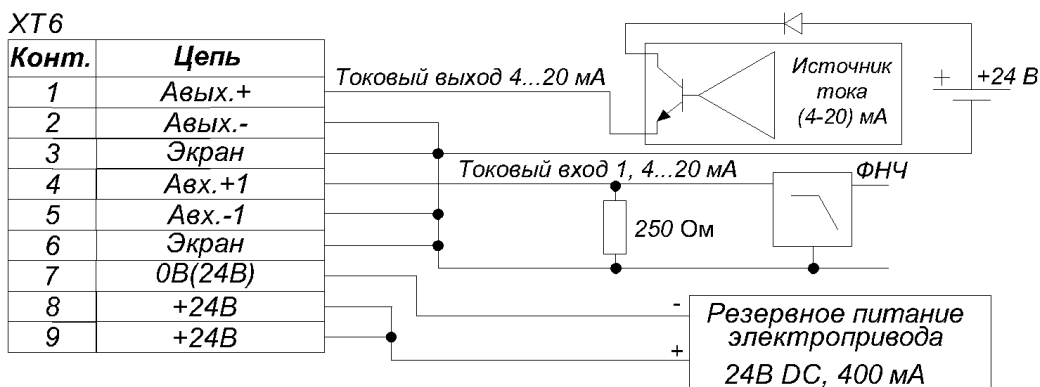
Рисунок 22 – Схема подключения
