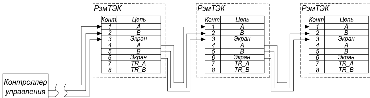
Рисунок 16 – Схема 2
