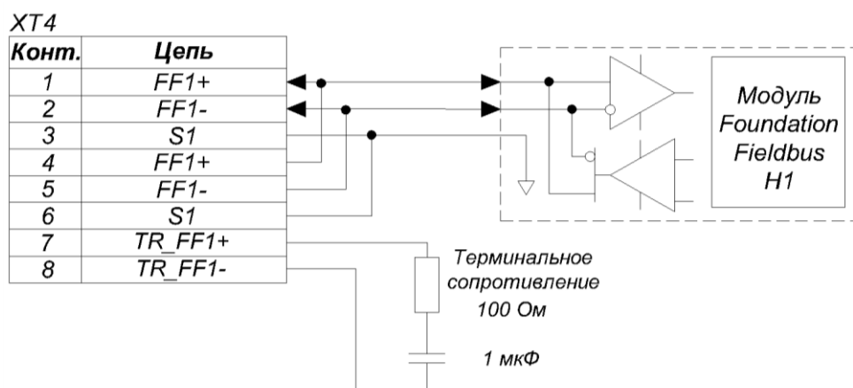
Рисунок 20 – Структурная схема подключения интерфейса Foundation Fieldbus
