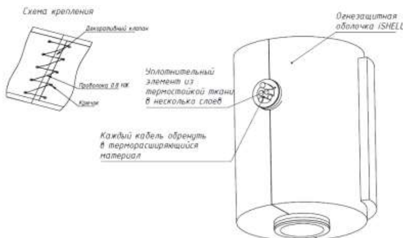
Рисунок 38 – Схема 2
