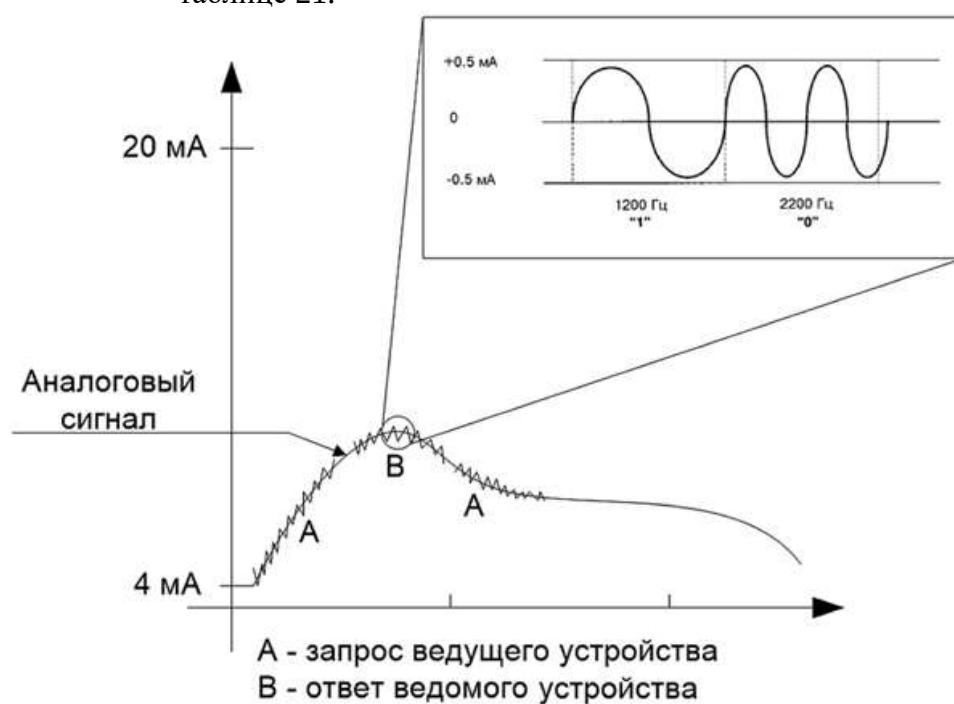
Рисунок 20 – Кодирование HART-сигнала
