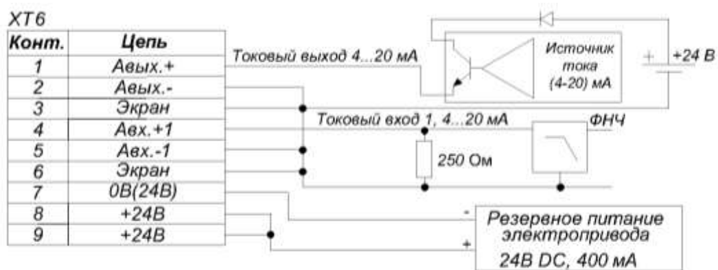
Рисунок 27 – Схема подключения
