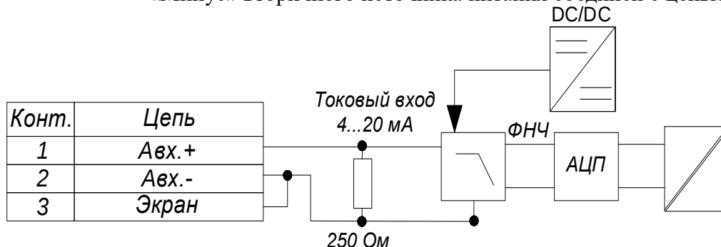
Рисунок 14 – Структурная схема аналогового входа
