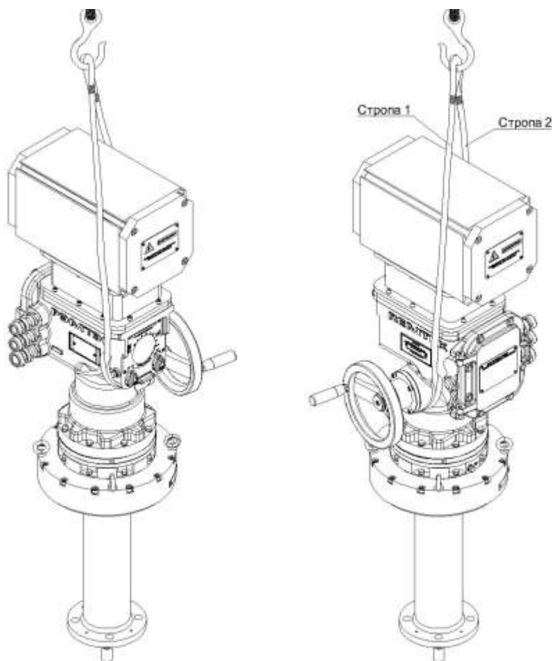
Рисунок 29 – Схемы строповки электропривода Л.65000.50 конструктивного исполнения «9400»
