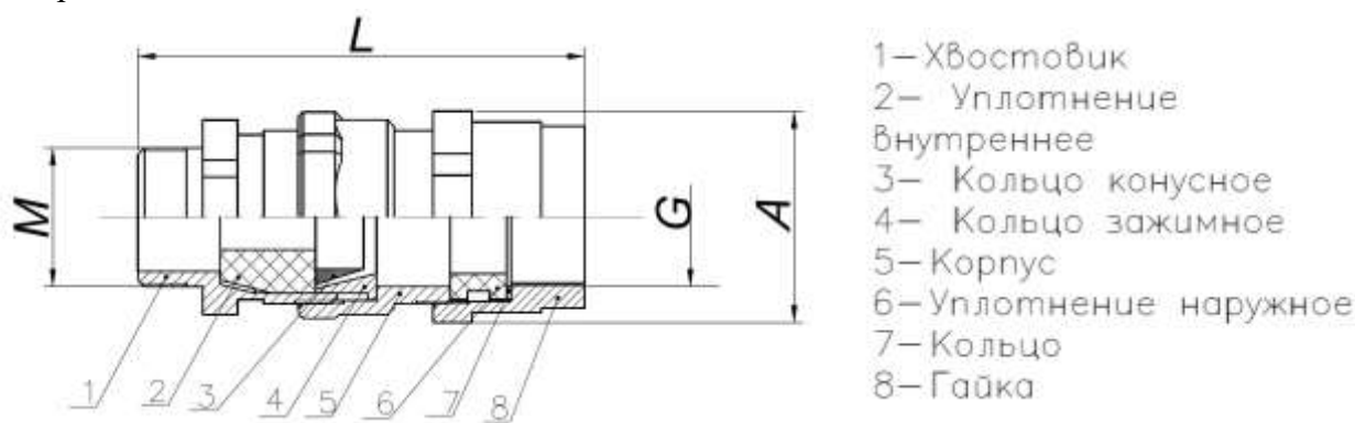
Рисунок Д.1 – Кабельный ввод ТАВВКу
