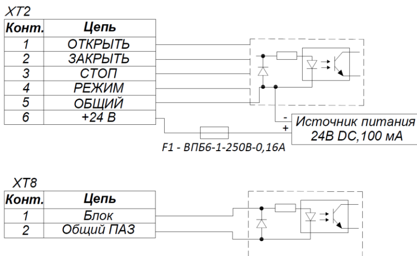
Рисунок 7 – Структурная схема дискретных входов
