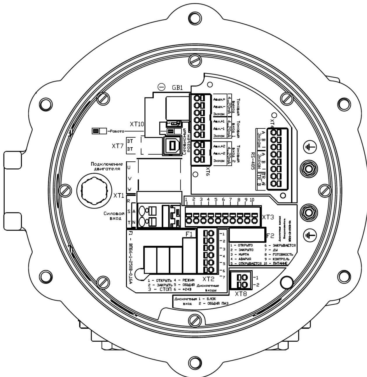
Рисунок 18а – Типовой внешний вид бокса РэмТЭК конструктивного исполнения «81»
