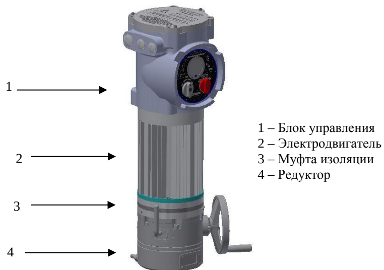
Рисунок 2 – Составные части электропривода РэмТЭК конструктивного исполнения «8»
