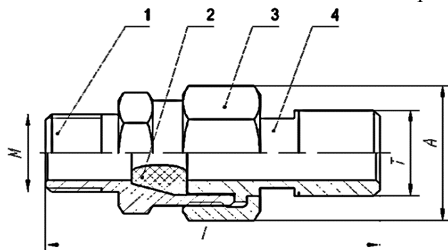
а) Кабельный ввод КВВ.р....
