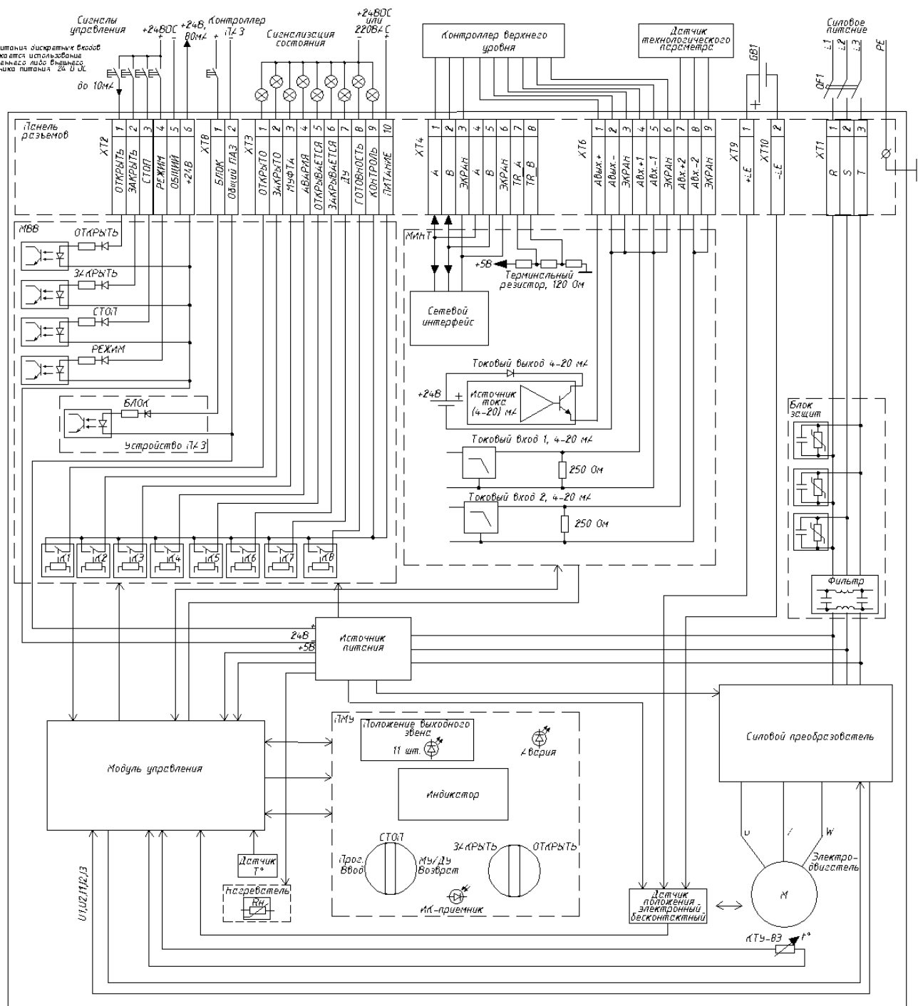
Рисунок И.2 – Схема электрическая функциональная РэмТЭК при питании от трехфазной цепи переменного тока напряжением 400 В или комбинированном питании напряжением 230/400 В частотой 50 Гц
