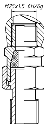
Рисунок В.1 – Типы кабельных вводов, используемых в РэмТЭК конструктивного исполнения "8"
