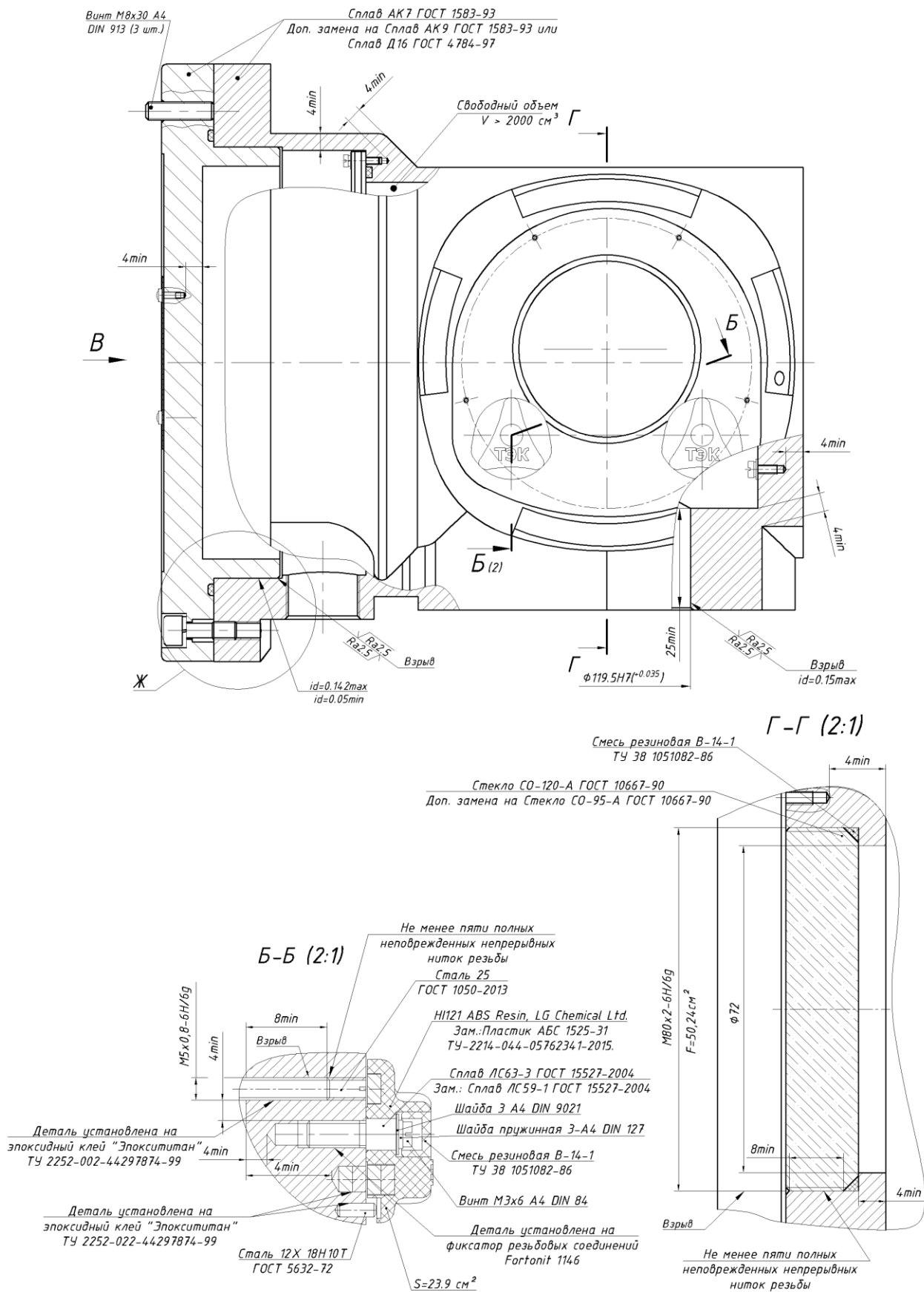
Рисунок Ж.6 – Чертеж средств взрывозащиты РэмТЭК конструктивного исполнения "82хх"
