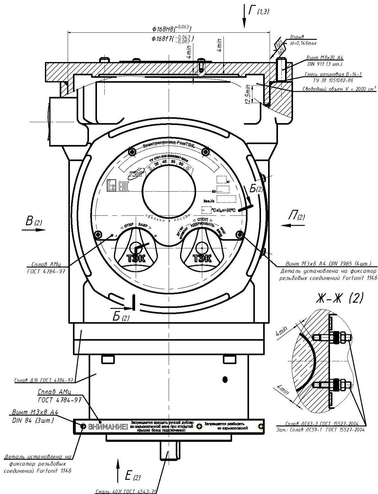
Рисунок Ж.4 – Чертеж средств взрывозащиты РэмТЭК конструктивного исполнения "80х2" с питанием 400 В
