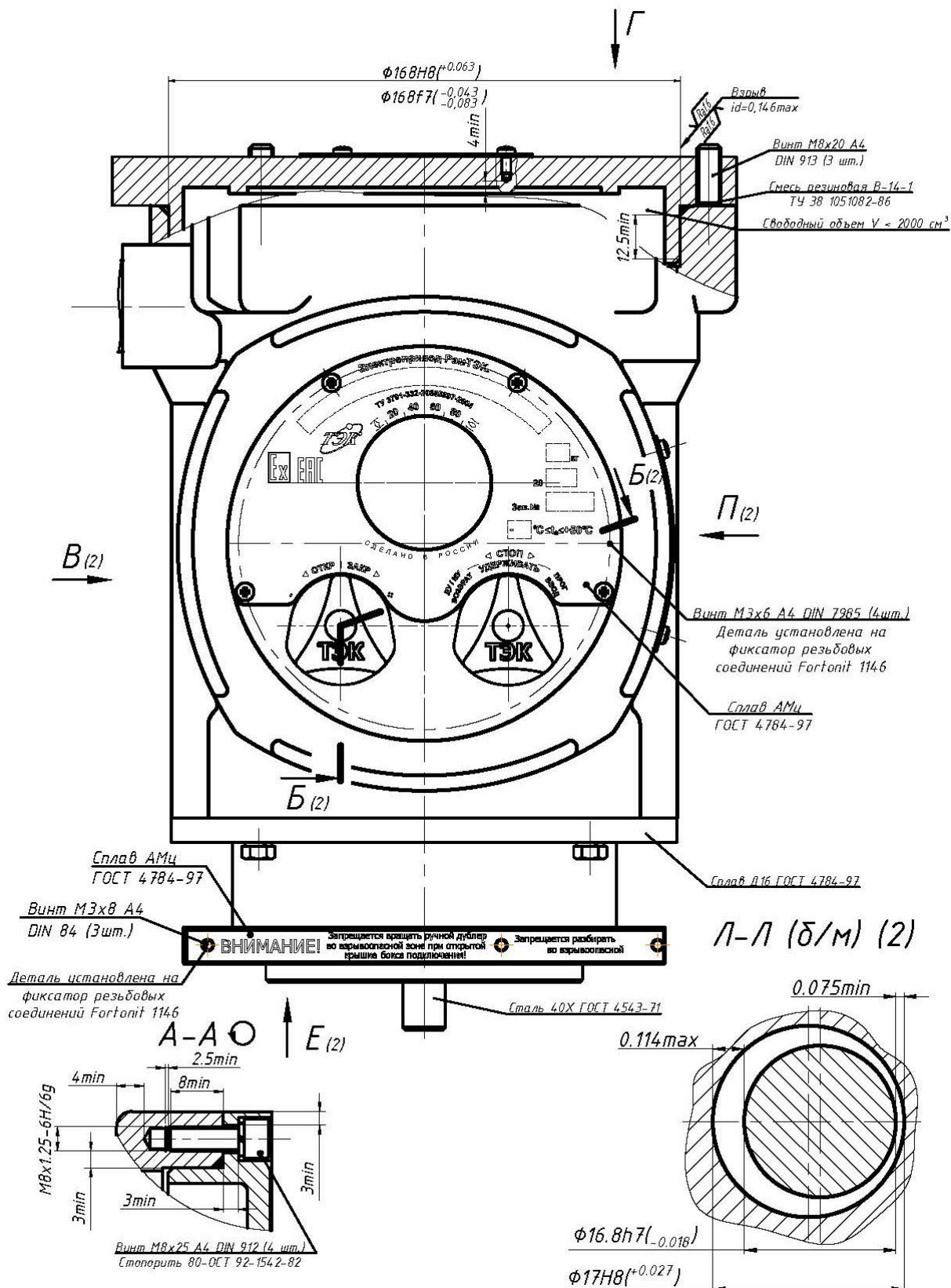
Рисунок Ж.3 – Чертеж средств взрывозащиты РэмТЭК конструктивного исполнения "80х2" с питанием 230 В
