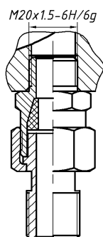
Рисунок В.1 – Типы кабельных вводов, используемых в РэмТЭК конструктивного исполнения "8"
