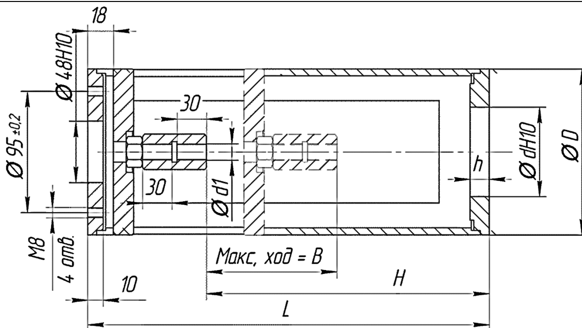
Рисунок В.3 – Присоединительное звено прямоходных РэмТЭК к арматуре
