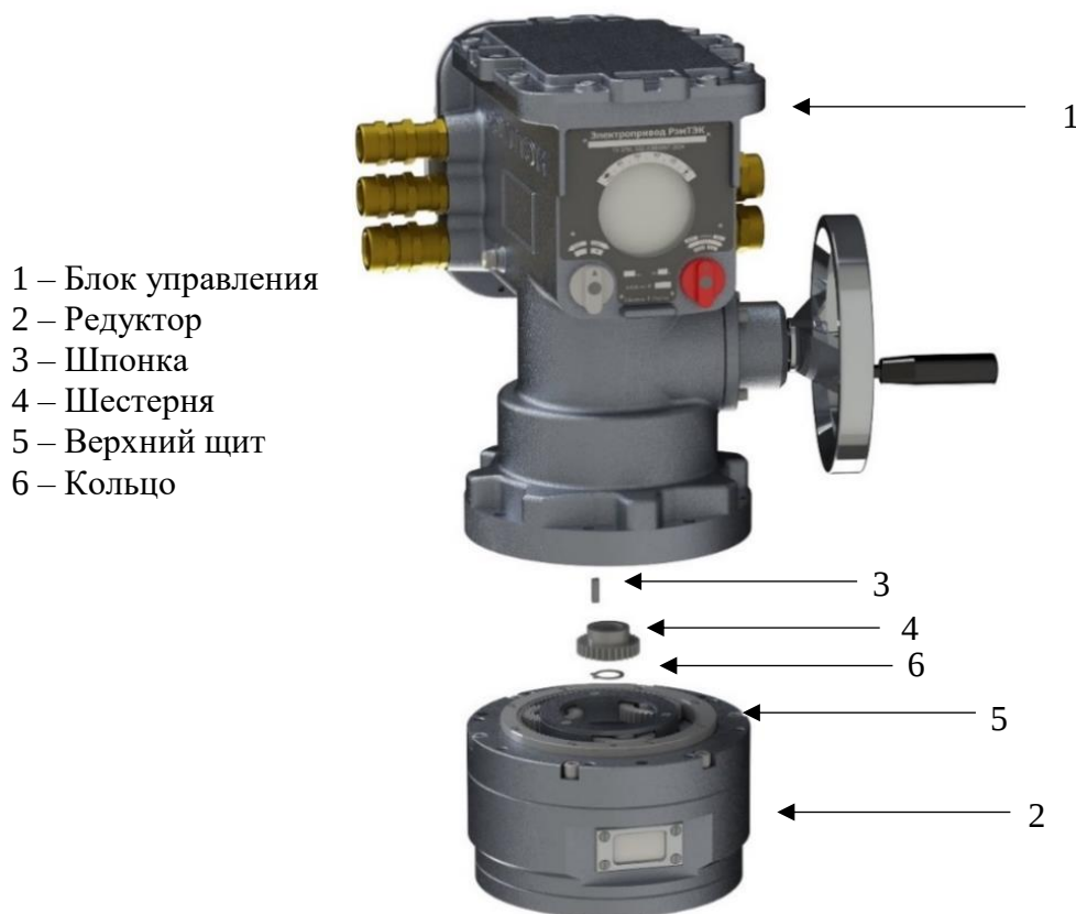
Рисунок 29 – Порядок замены редуктора
