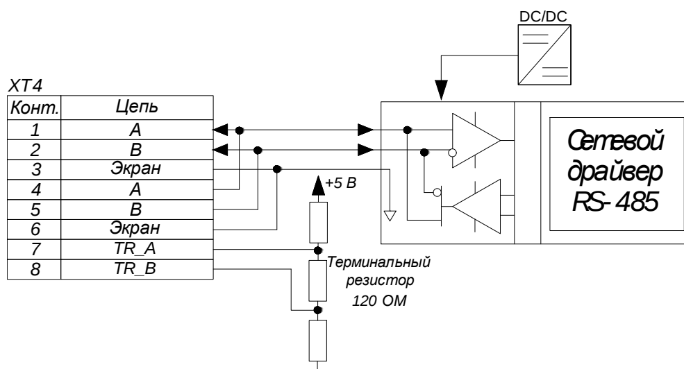
Рисунок 13 – Структурная схема RS-485
