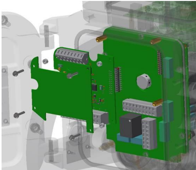
Рисунок 31 - Замена МИНТ
