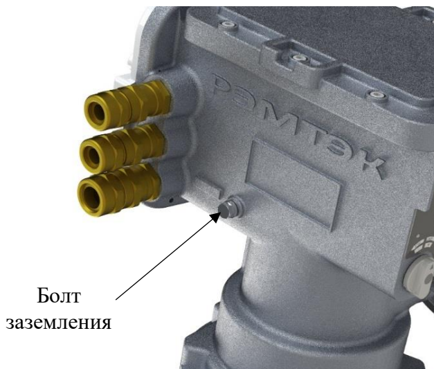
Рисунок 20 – Заземление электропривода
