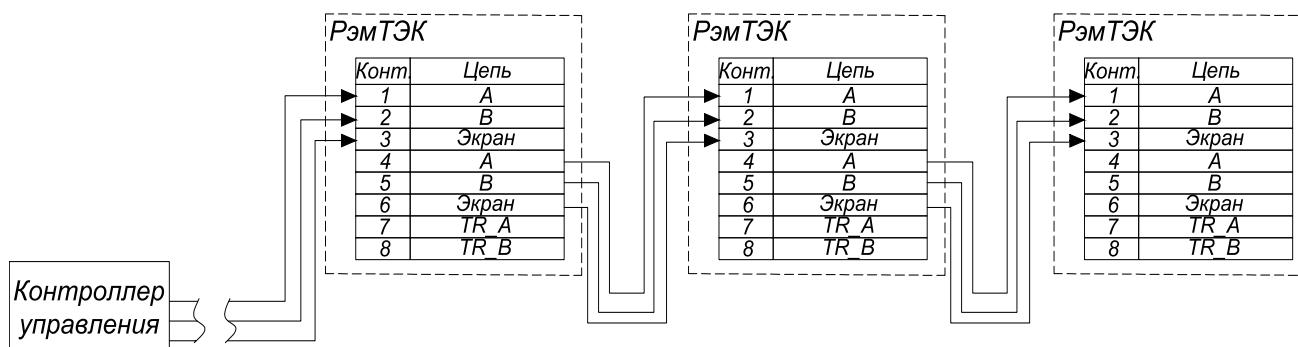
Рисунок 15 – Схема 2
