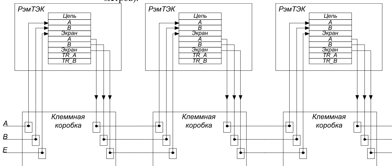
Рисунок 14 – Схема 1
