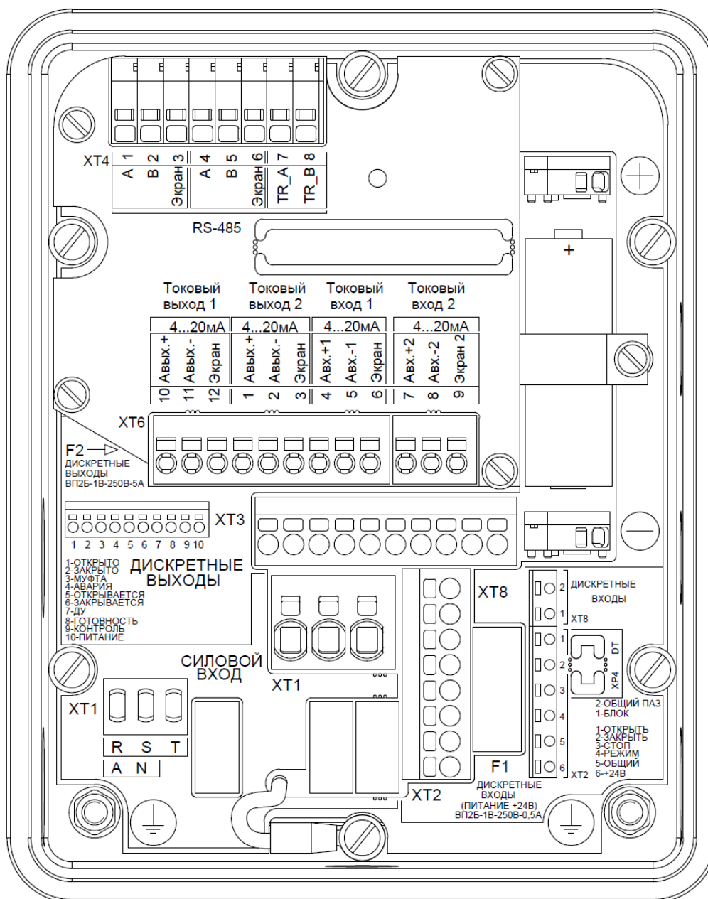
Рисунок 22 – Внешний вид бокса подключения
