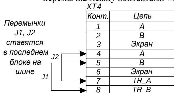
Рисунок 15а – Схема подключения с помощью перемычек
