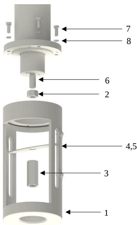
Рисунок 18 – Схема установки РэмТЭК прямоходного исполнения
