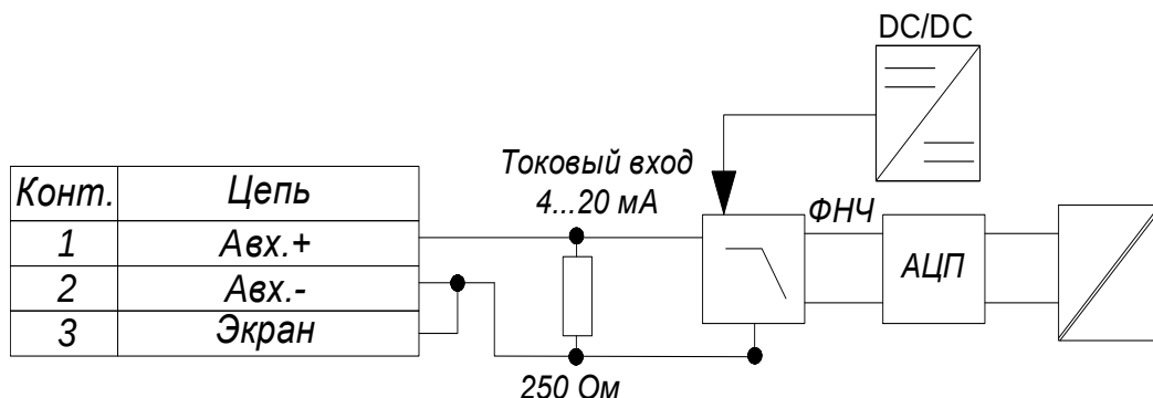
Рисунок 11 – Структурная схема аналогового входа
