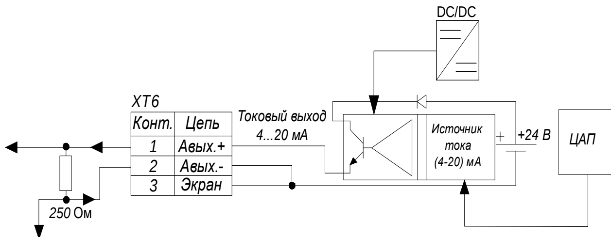
Рисунок 12 – Структурная схема аналогового выхода
