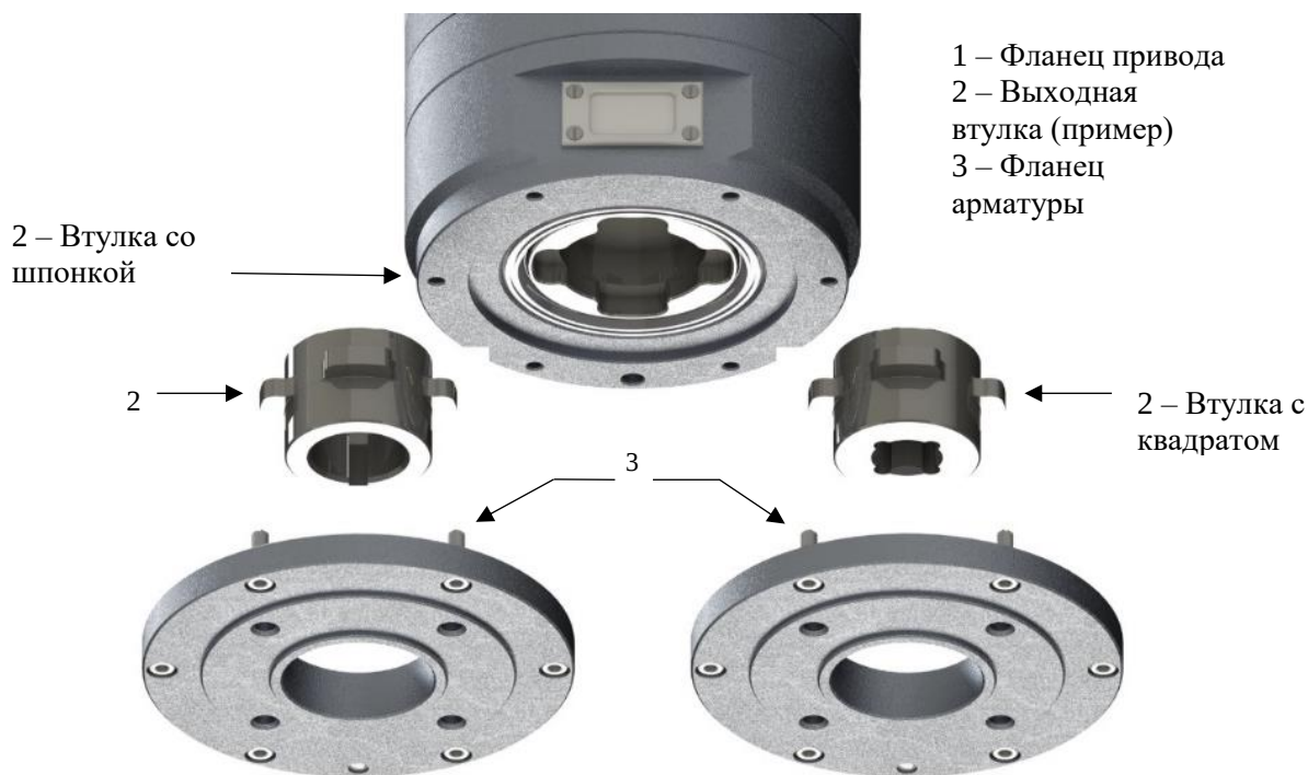
Рисунок 17 – Схема установки РэмТЭК многооборотного и неполнооборотного исполнения
