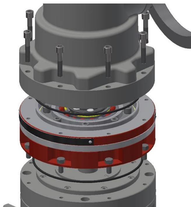
Рисунок 30 – Порядок замены редуктора
