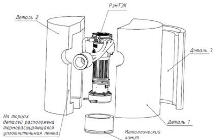
Рисунок 22б – Схема 1
