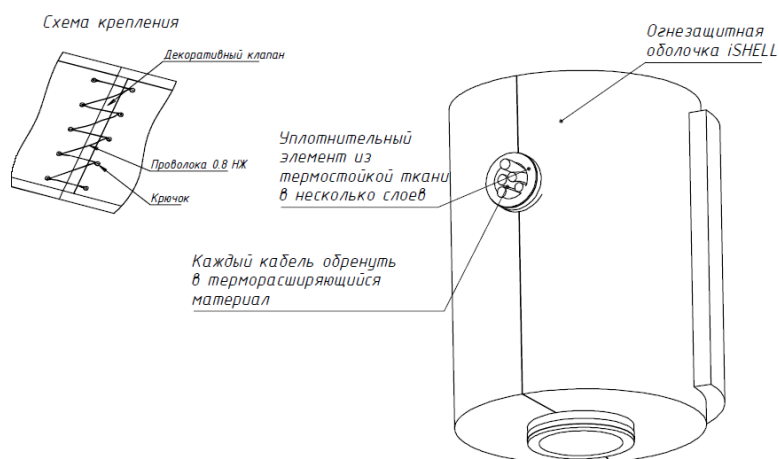
Рисунок 22в – Схема 2
