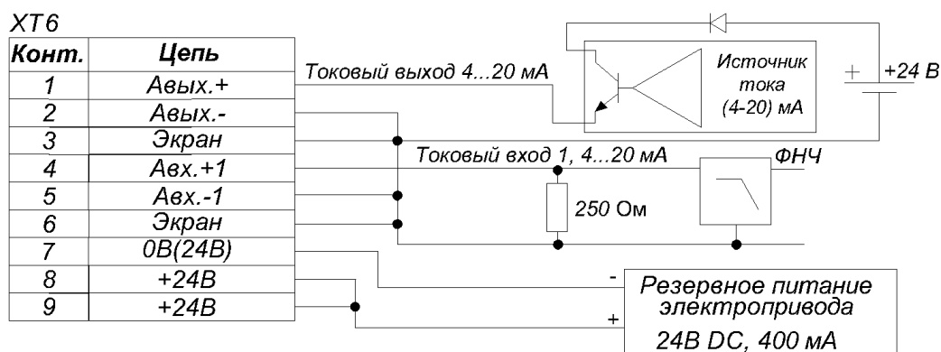
Рисунок 15г – Схема подключения
