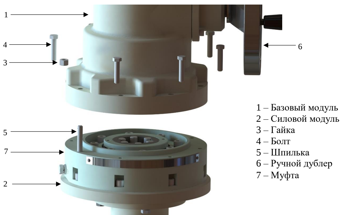
Рисунок 19 – Поворот БМ относительно редуктора
