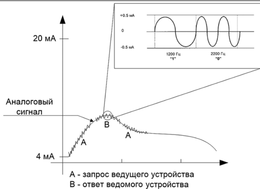
Рисунок 15б – Кодирование HART-сигнала
