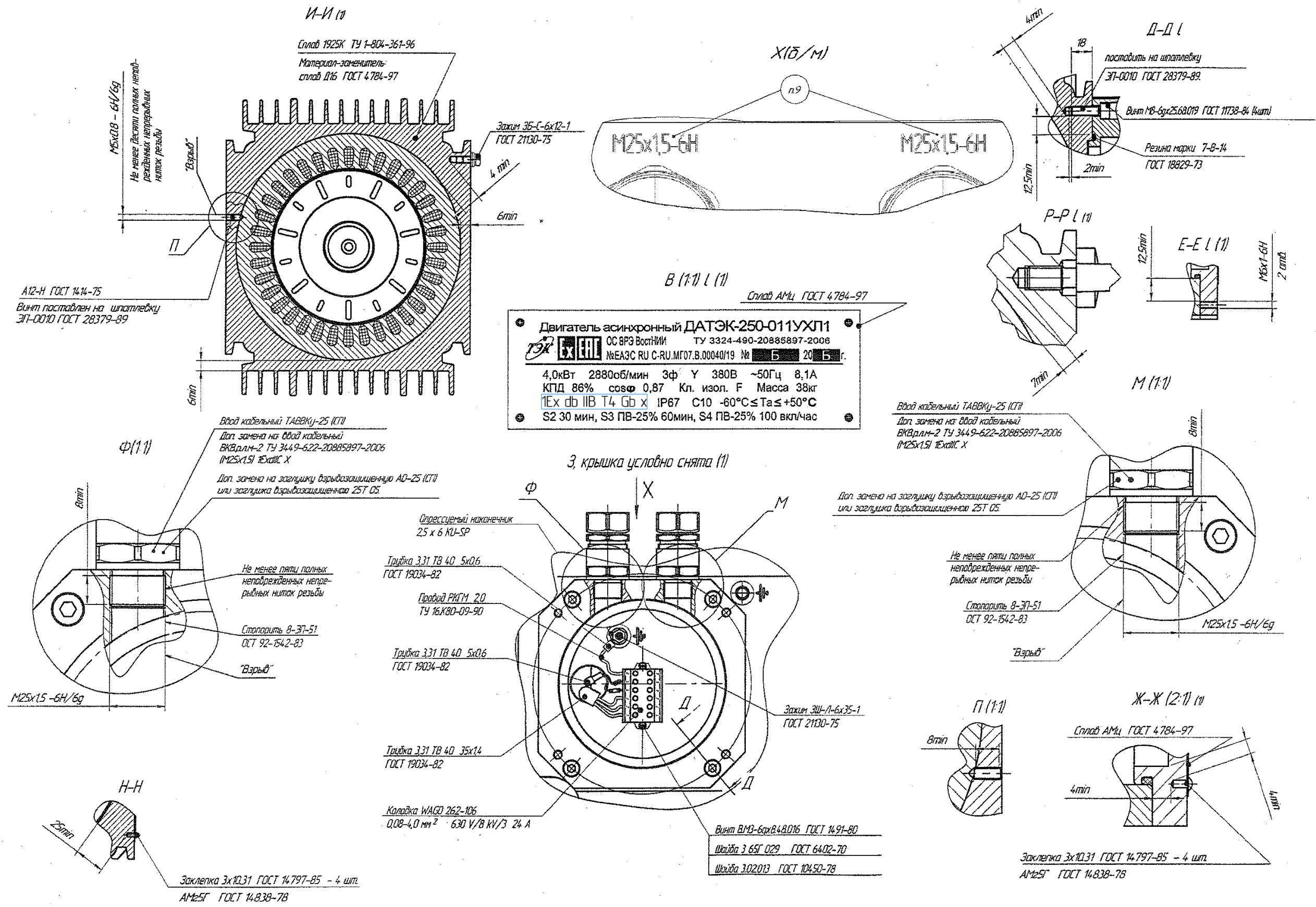
Рисунок В.1 – Чертеж средств взрывозащиты для модификации ДАТЭК-250-XX0, ДАТЭК-250-XX1, ДАТЭК-250-XX3 и ДАТЭК-250-XX4 (лист 2 из 4)
