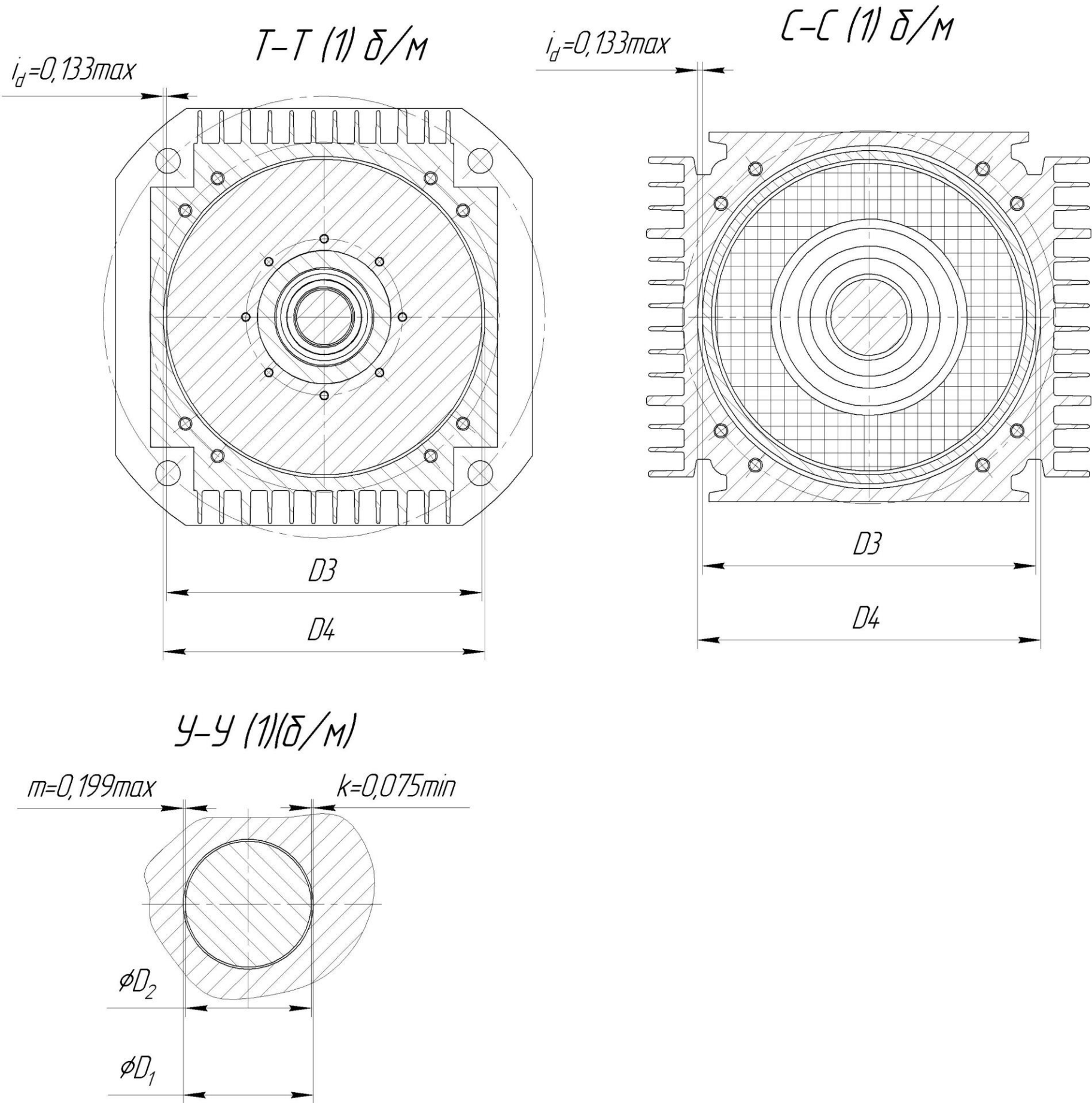
Рисунок В.1 – Чертёж средств взрывозащиты для модификации ДАТЭК-250-XX0, ДАТЭК-250-XX1, ДАТЭК-250-XX3 и ДАТЭК-250-XX4 (лист 3 из 4)
