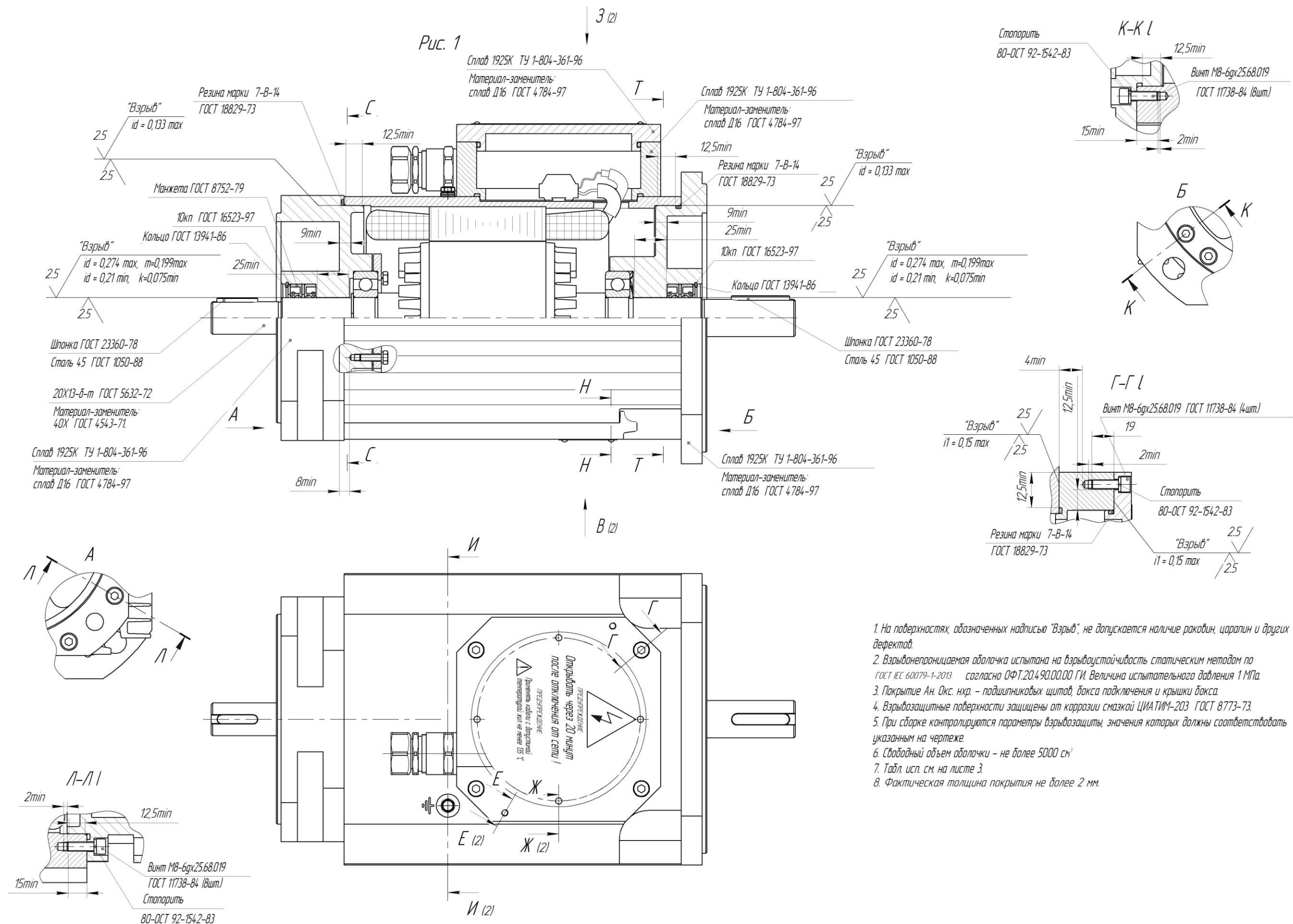
Рисунок В.2 – Чертёж средств взрывозащиты для модификации ДАТЭК-250-XX2, ДАТЭК-250-XX5 (лист 1 из 4)
