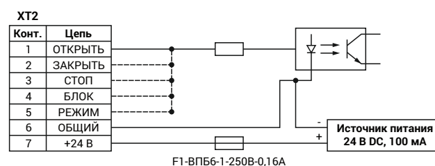
Структурная схема дискретного входа
