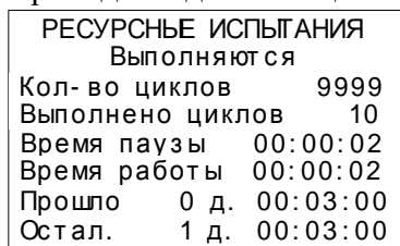
Рисунок 14 – Экран текущих параметров ресурсных испытаний
