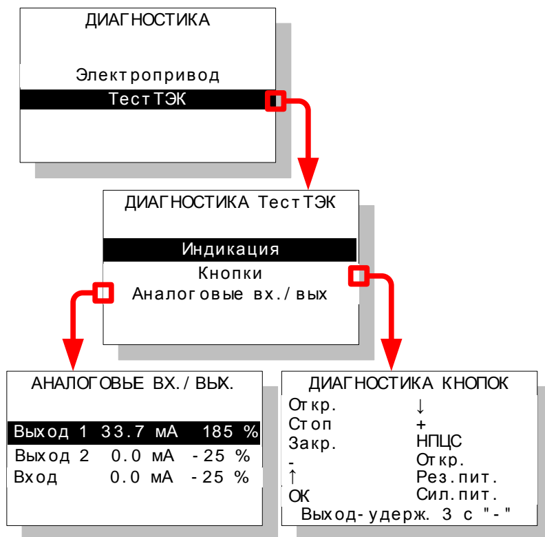
Рисунок 15 – Меню диагностики ТестТЭК.
