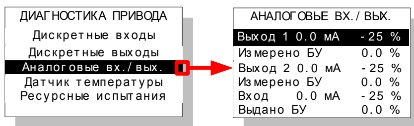
Рисунок 11 – Подменю тестирования аналоговых входов и выходов
