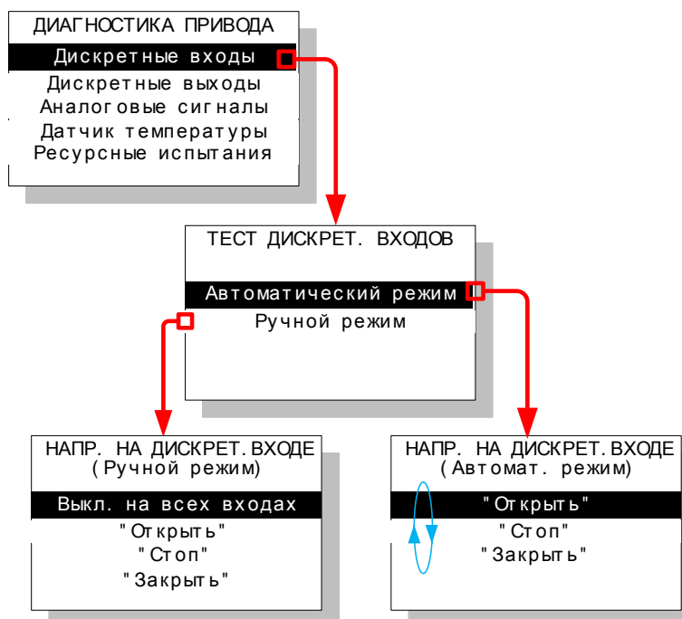
Рисунок 9 – Структура подменю "Диагностика привода"–
